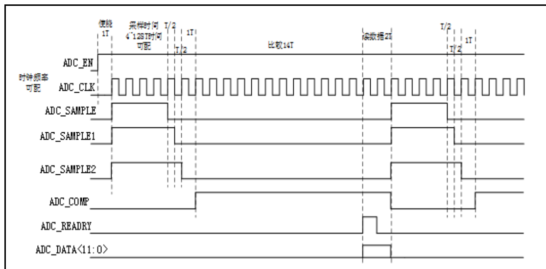
图 10-8 ADC 时序图
