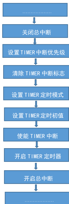
TIMER 配置流程图
