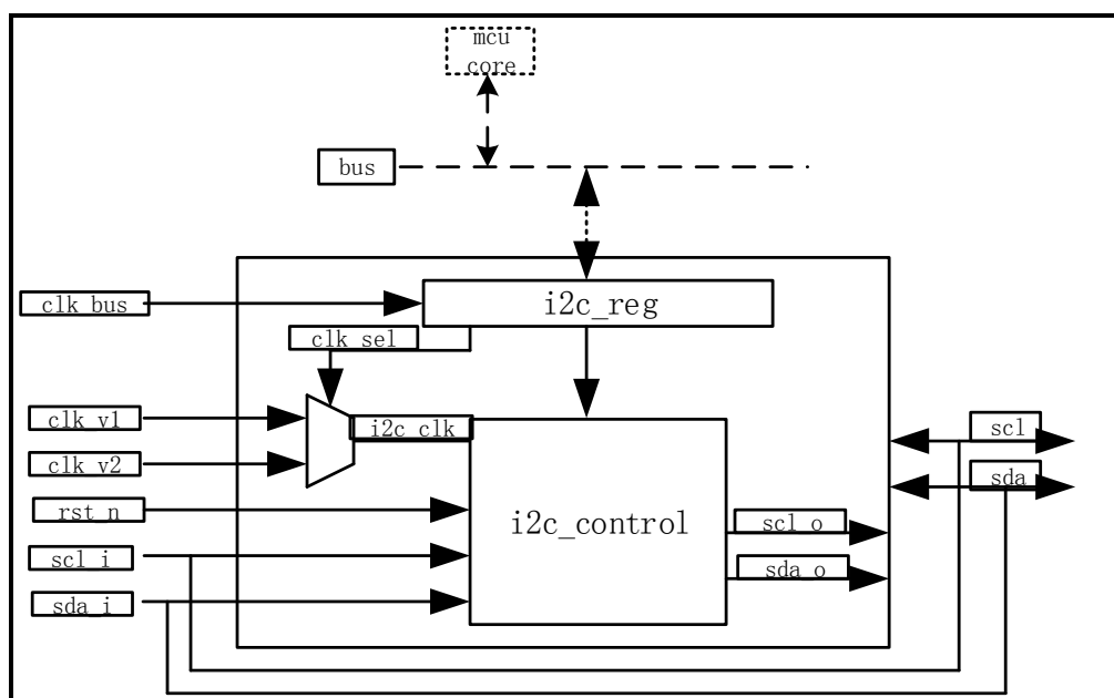
图 10-10 I2C 结构框图
