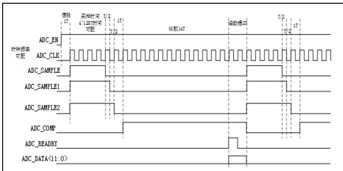
图 10-8 ADC 时序图
