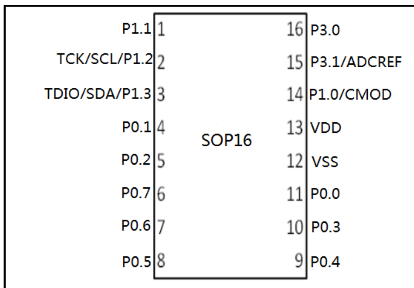
图 4-8 SOP16 封装脚位图(支持引脚功能全映射)
