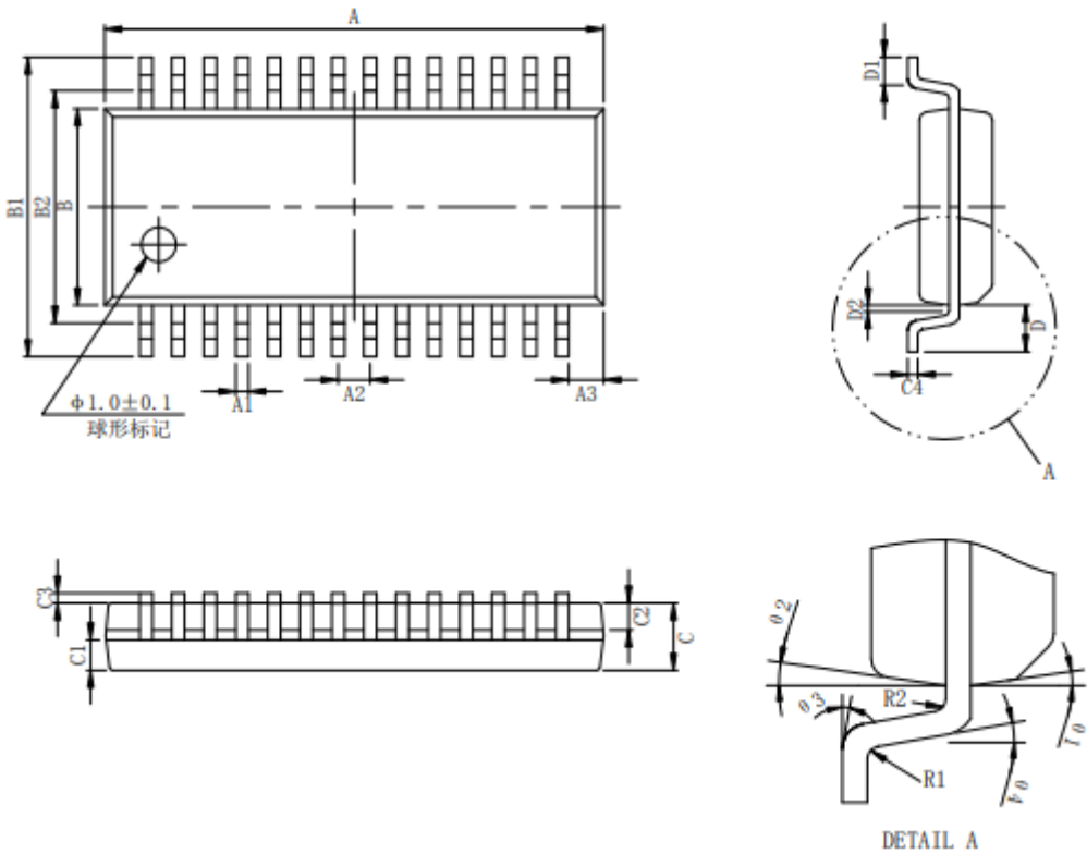
图 16-1 SS0P28 封装外形图
