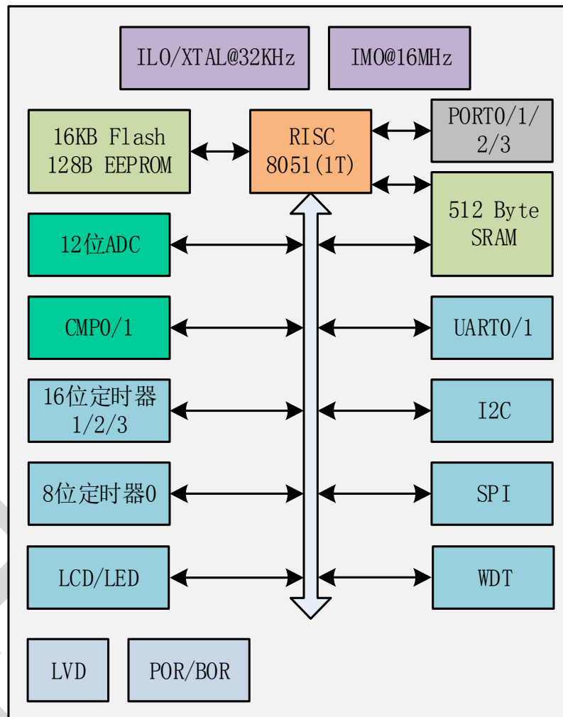
图 3-1 结构框图
