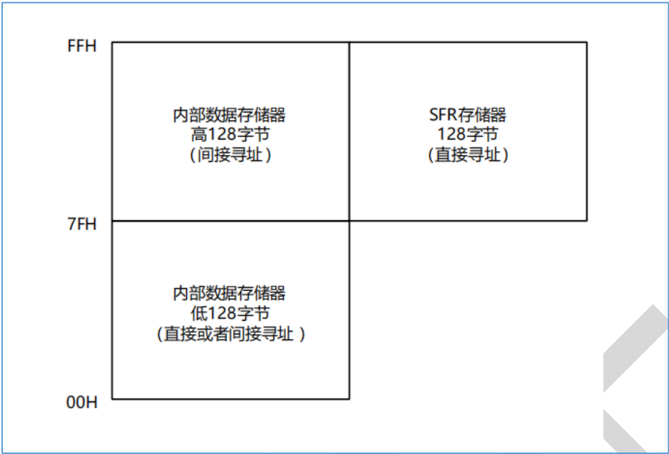
图 6-2 数据存储器
