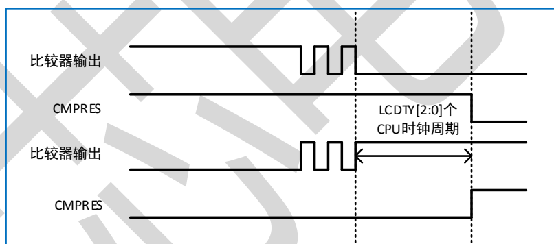
图 10-21 比较器数字滤波功能
