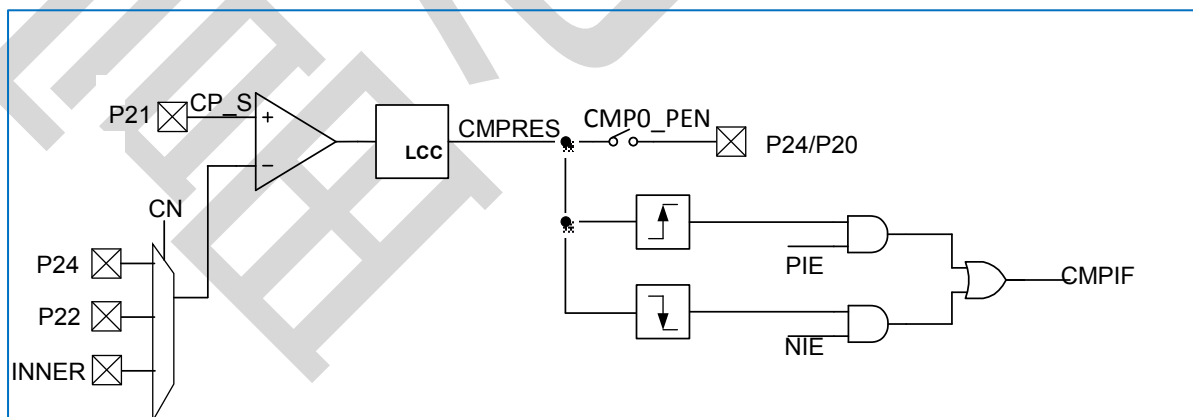
图 10-19 比较器 0 电路结构框图
