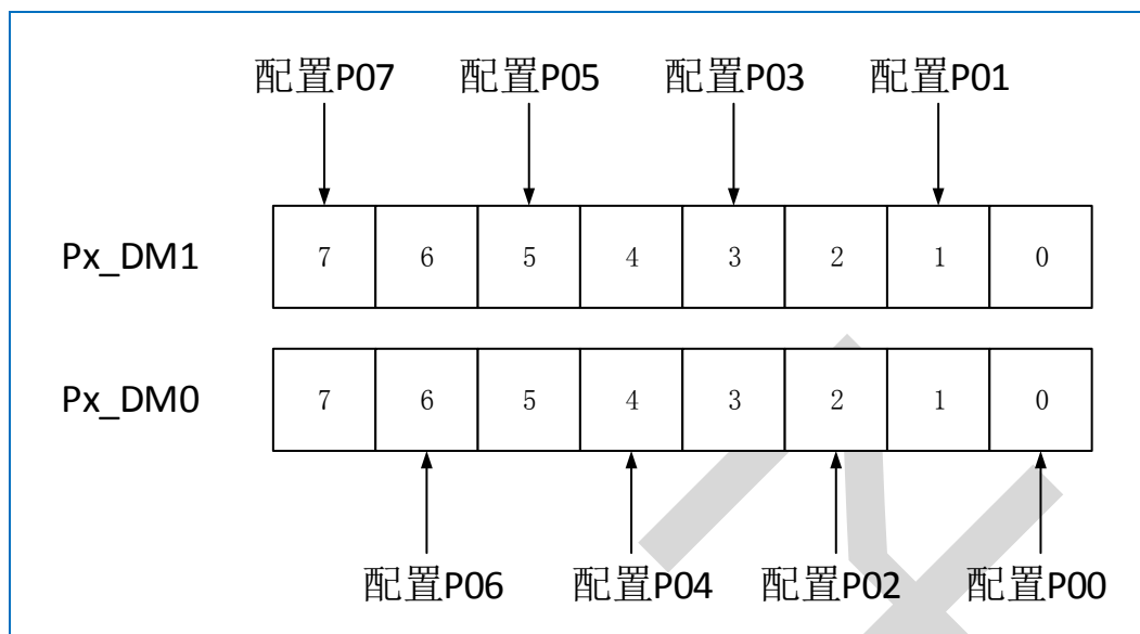
图 4-2 I/O 配置图
