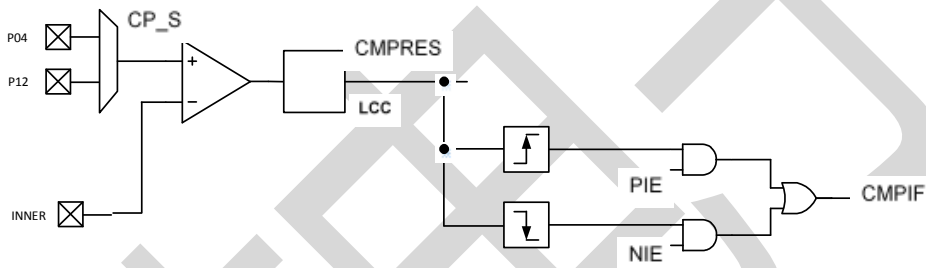
图 10-17 比较器 1 结构框图
