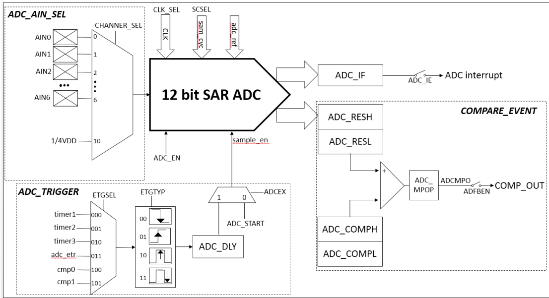
图 10-15 ADC 结构框图
