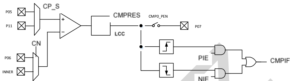
图 10-16 比较器 0 电路结构框图
