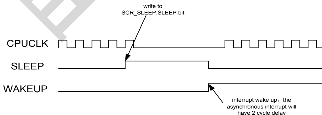
图 11-1 睡眠模式休眠和唤醒时序图
