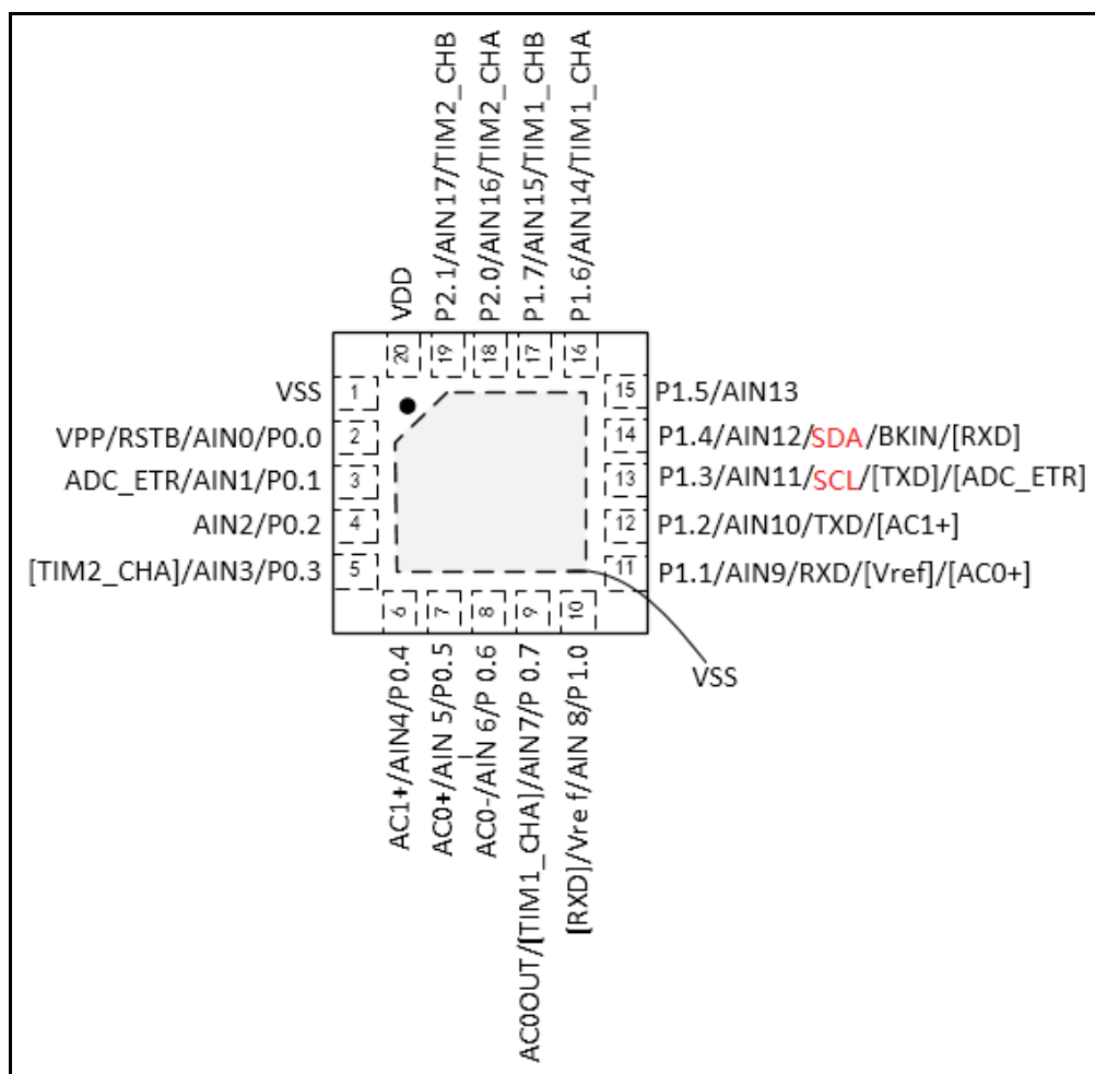
图 3-5 RC6F80042EB (QFN20) 引脚图
