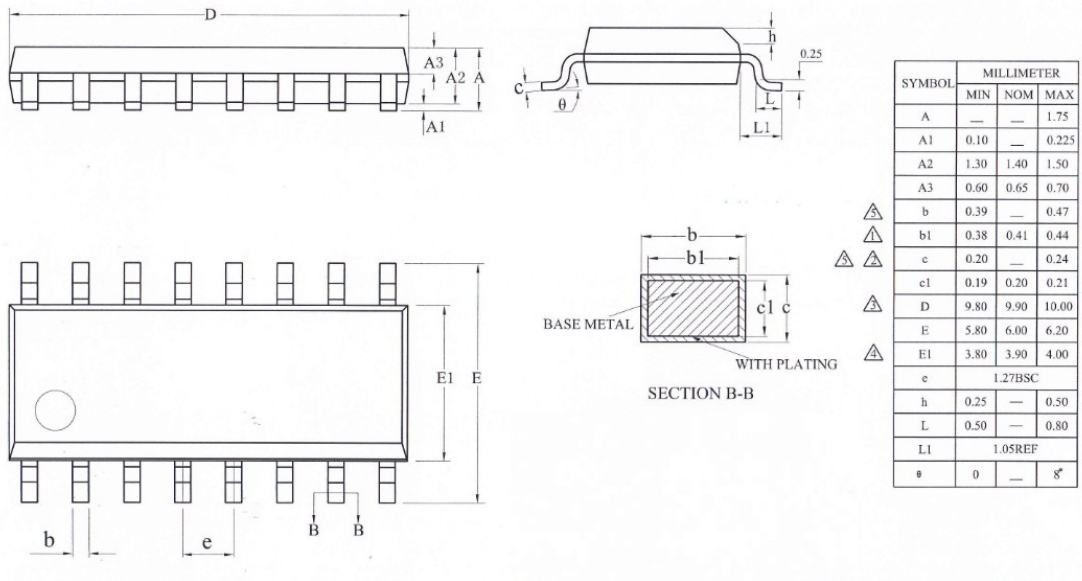
图 15-2 SOP16 封装外形图
