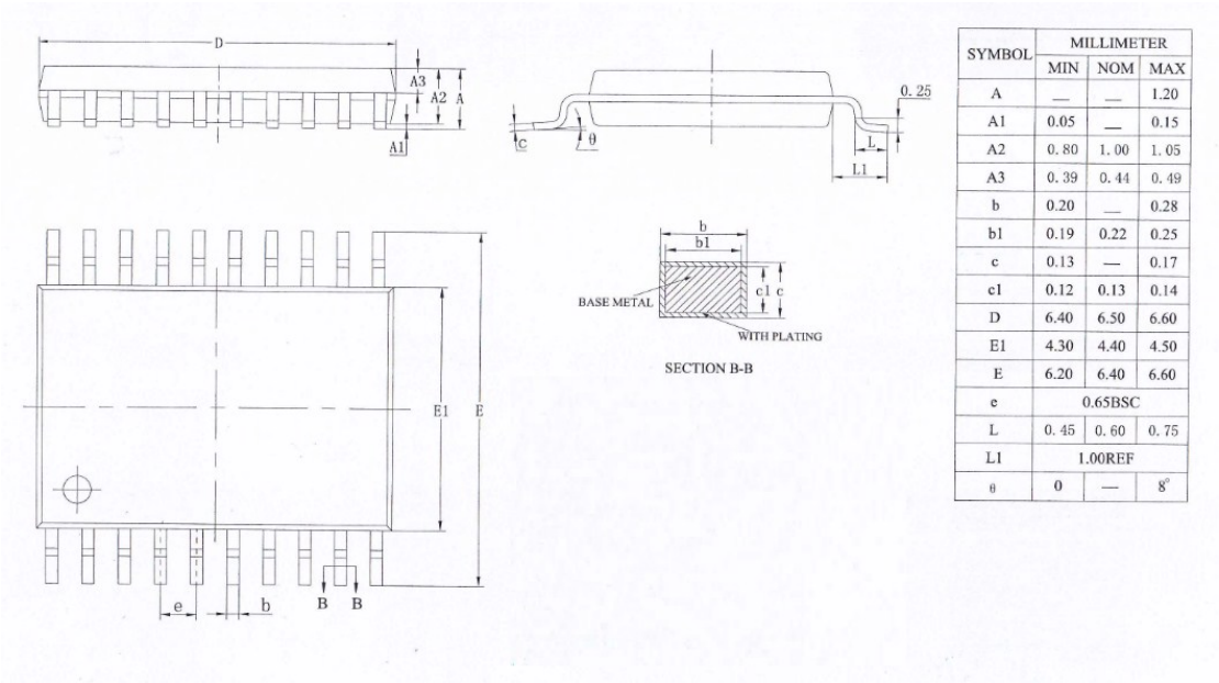
图 15-1 TSSOP20 封装外形图
