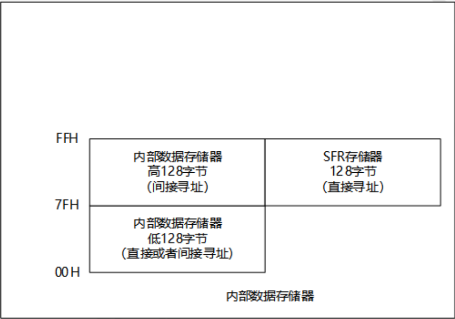
图 6-2 数据存储器
