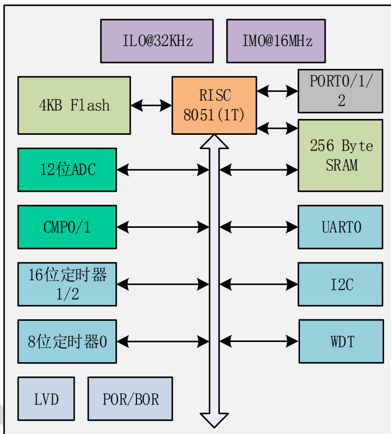
图 3-1 系统功能结构框图
