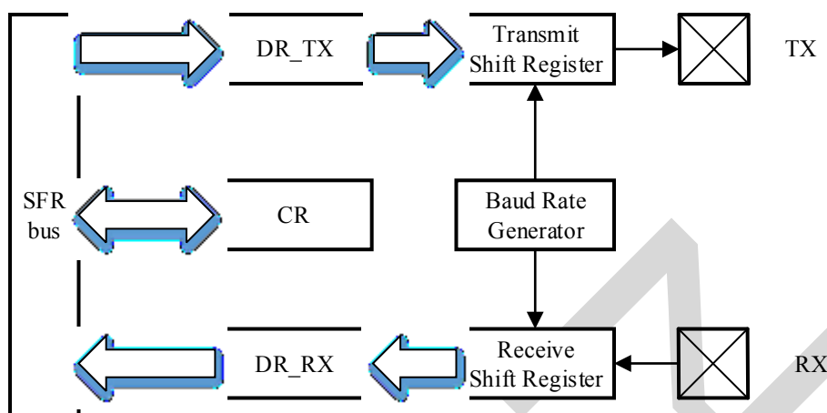
图 10-13 UART 结构框图
