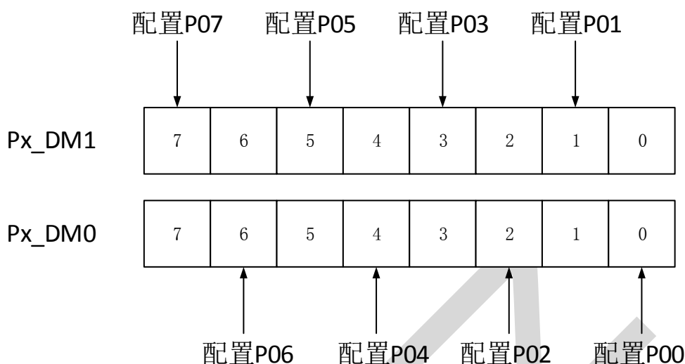
图 4-2 I/O 配置图
