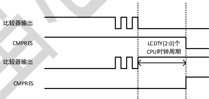
图 10-18 比较器数字滤波功能
