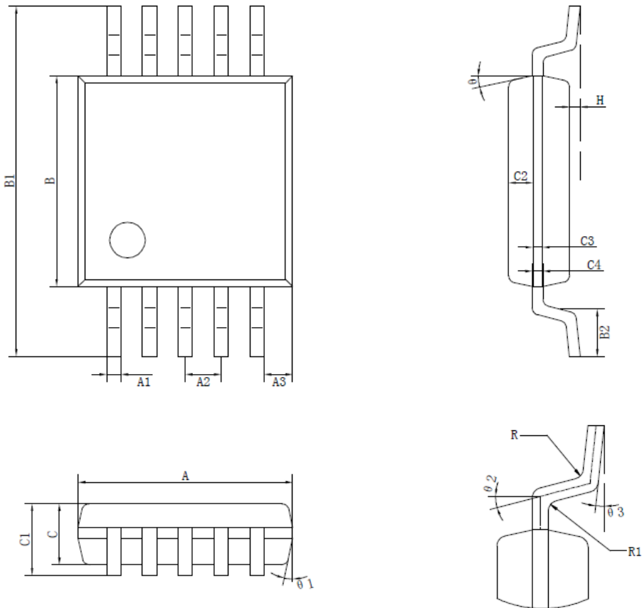
图 15-4 MSOP10 封装外形图
