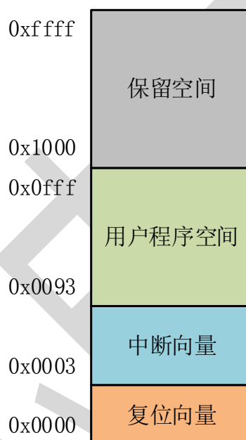
图 6-1 程序存储空间
