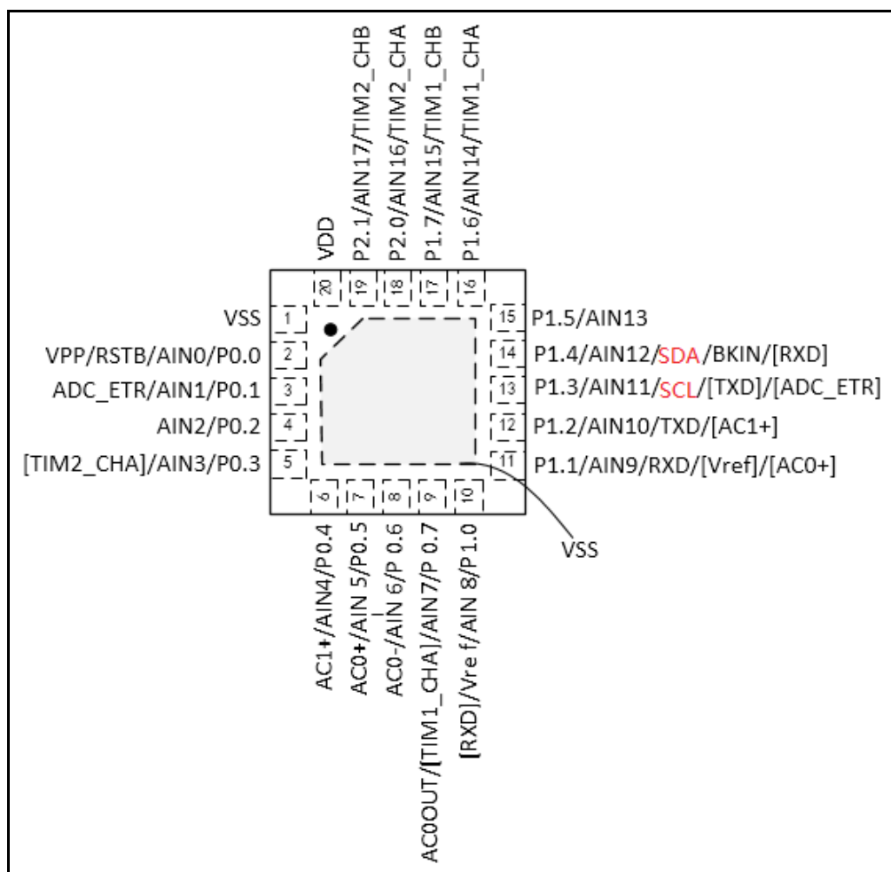
图 3-5 RC6F80042EB (QFN20) 引脚图
