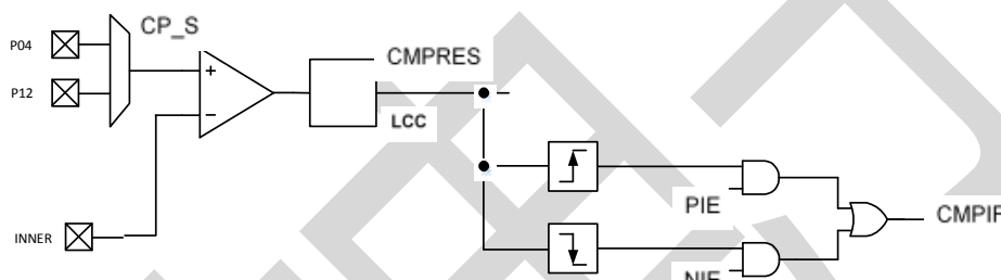
图 10-17 比较器 1 结构框图
