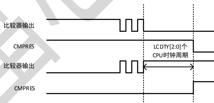
图 10-18 比较器数字滤波功能
