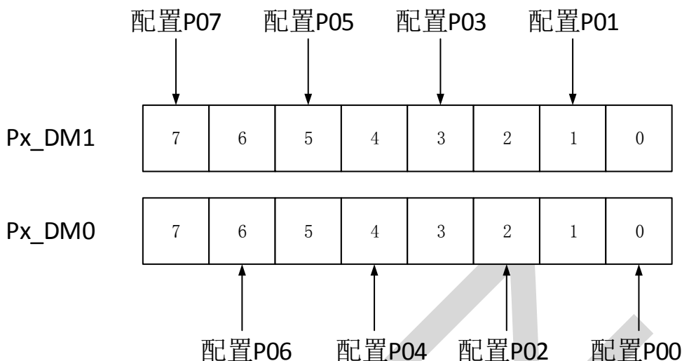
图 4-2 I/O 配置图
