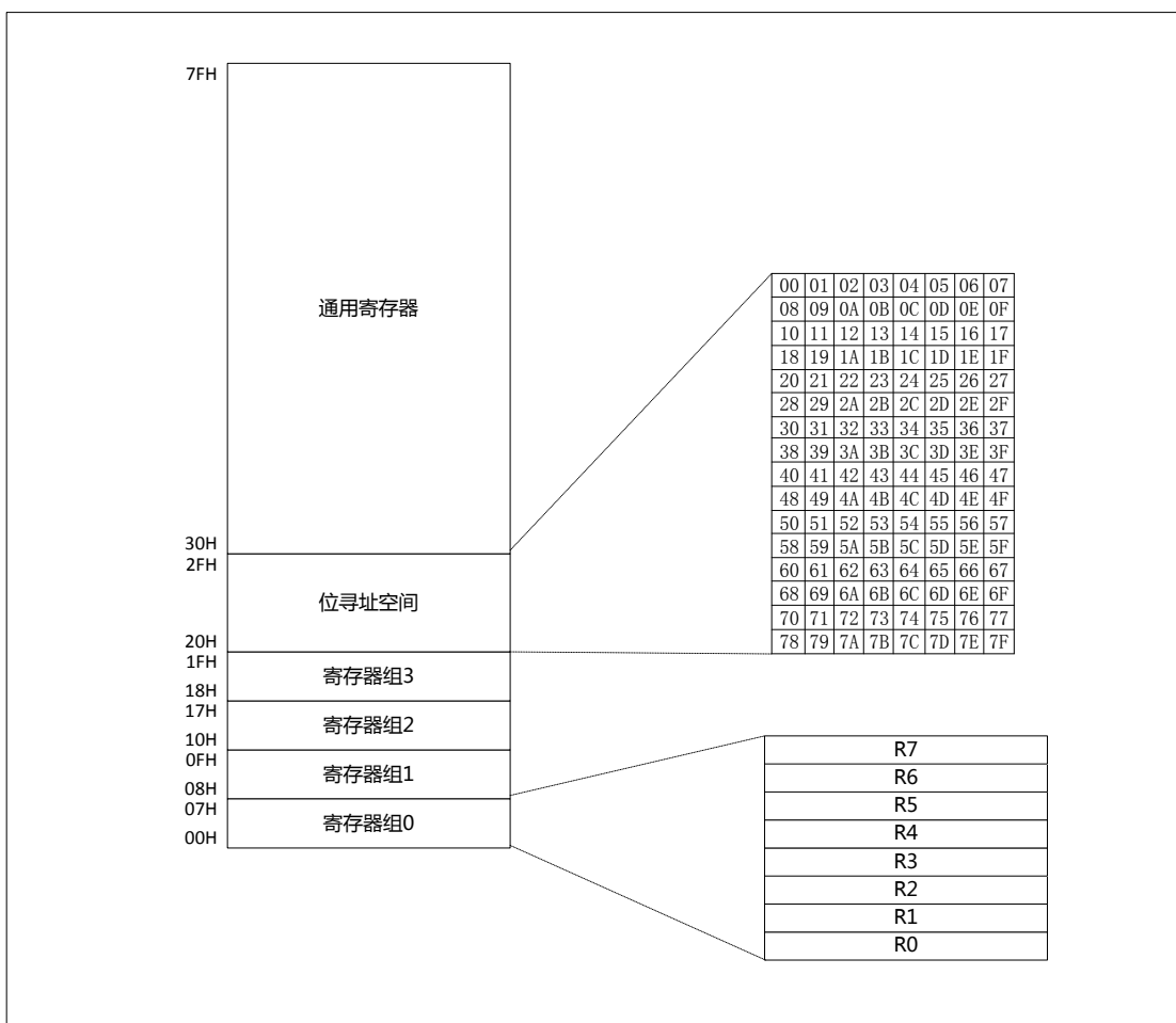
图 3-3 内部低 128 字节数据空间映射
