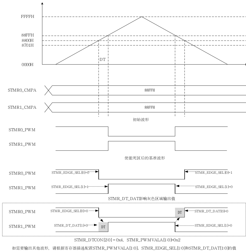
图 16-11 死区模式 4 互补波形图
