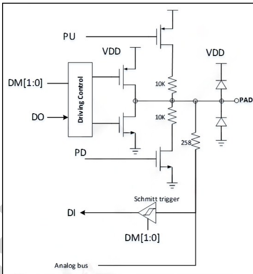
图 4-1 GPIO 结构图
