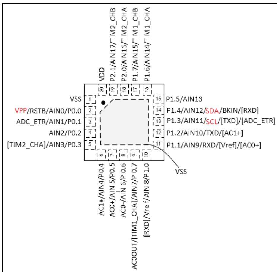
图 3-5 RC6F80042EB (QFN20) 引脚图
