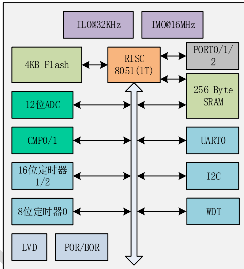
图 3-1 系统功能结构框图
