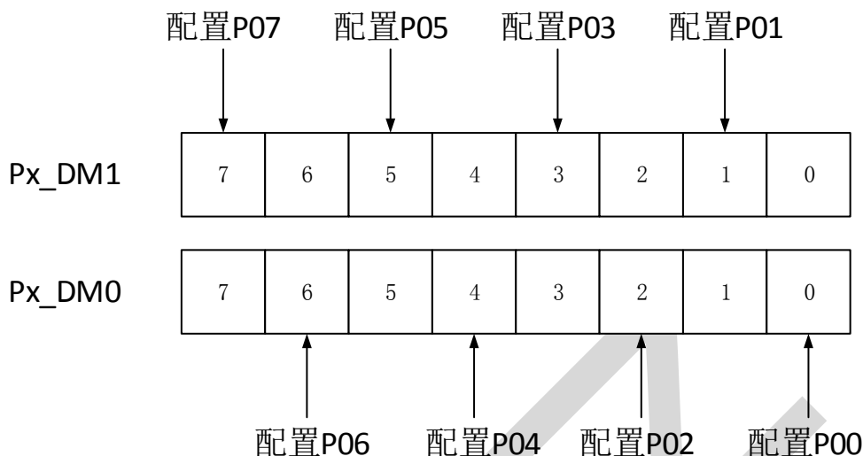
图 4-2 I/O 配置图
