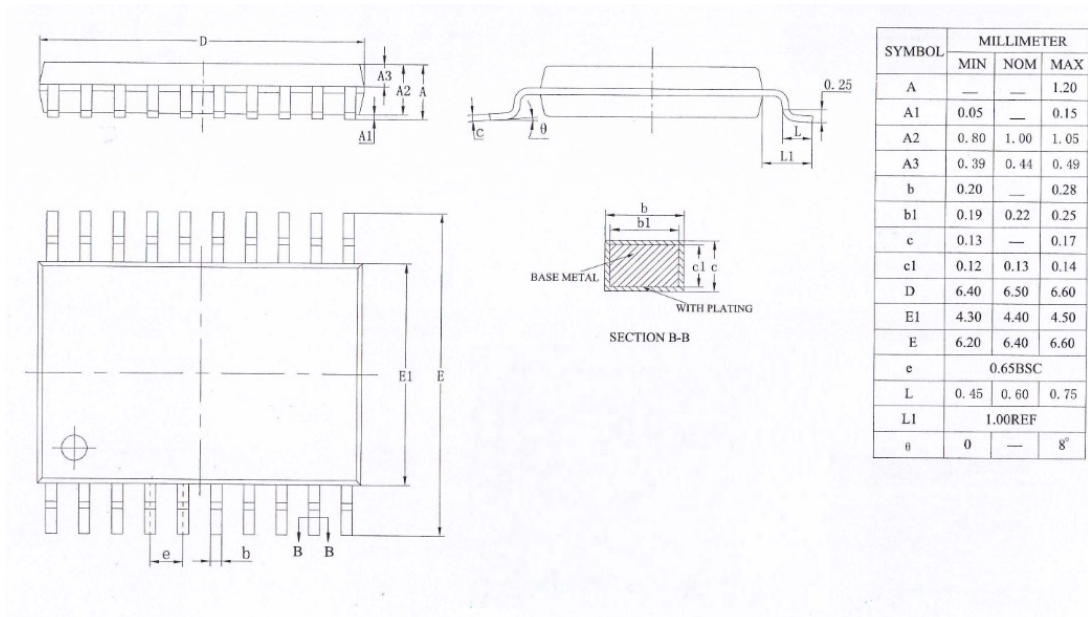
图 15-1 TSSOP20 封装外形图
