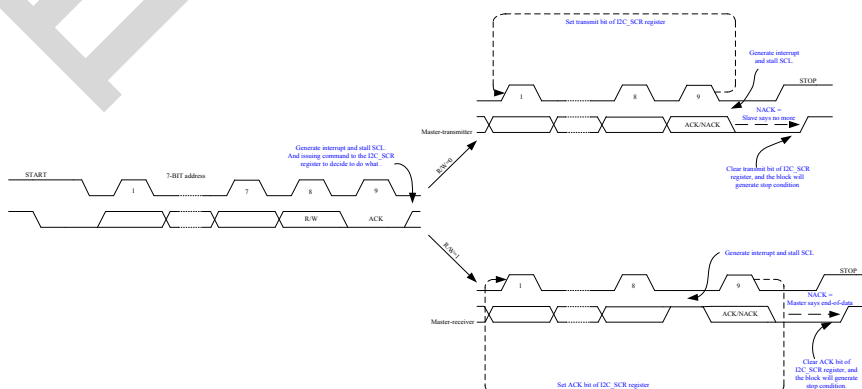
图 10-17 I2C 协议主机握手示意图 第 84 页 共 116 页
