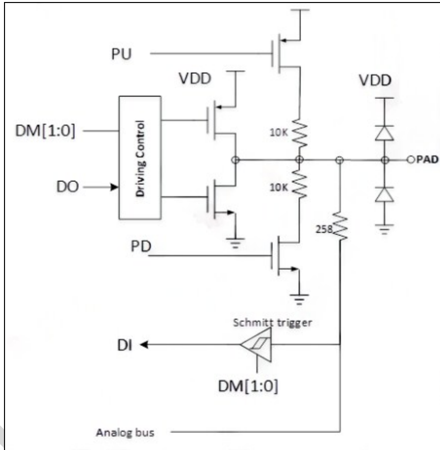
图 4-1 GPIO 结构图
