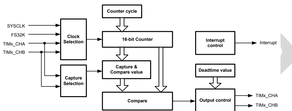
图 10-2 定时器结构图
