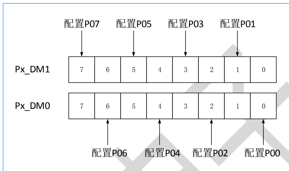
图 4-2 I/O 配置图
