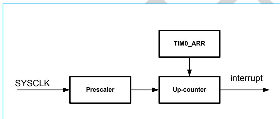
图 10-1 TIMERO 结构框图
