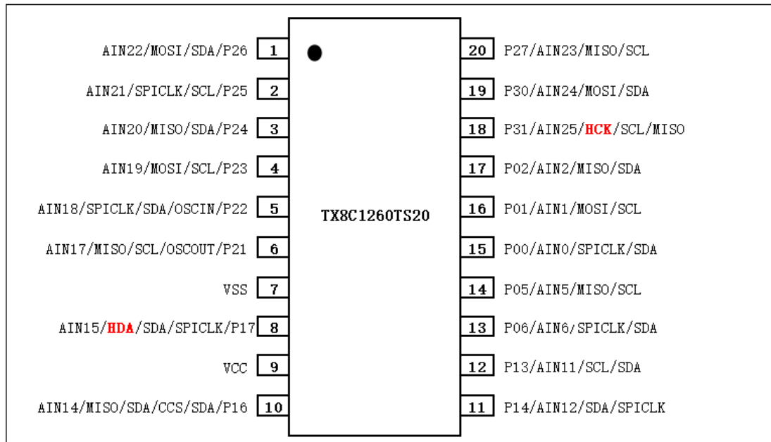
图 2 - TX8C1260TS20 (TSSOP20) 封装图
