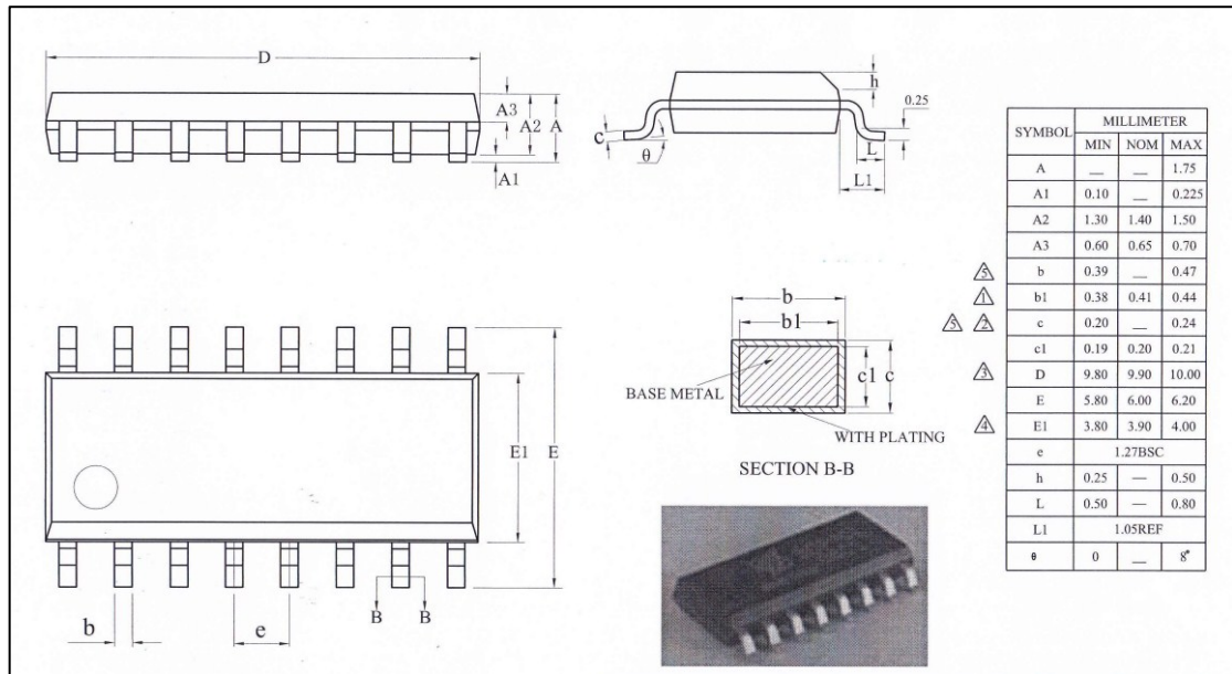
图 11- SOP16 封装 POD 图
