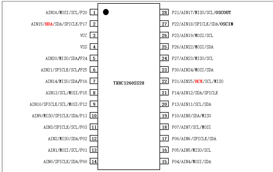
图 5 - TX8C1260SS28 (SSOP28) 封装图
