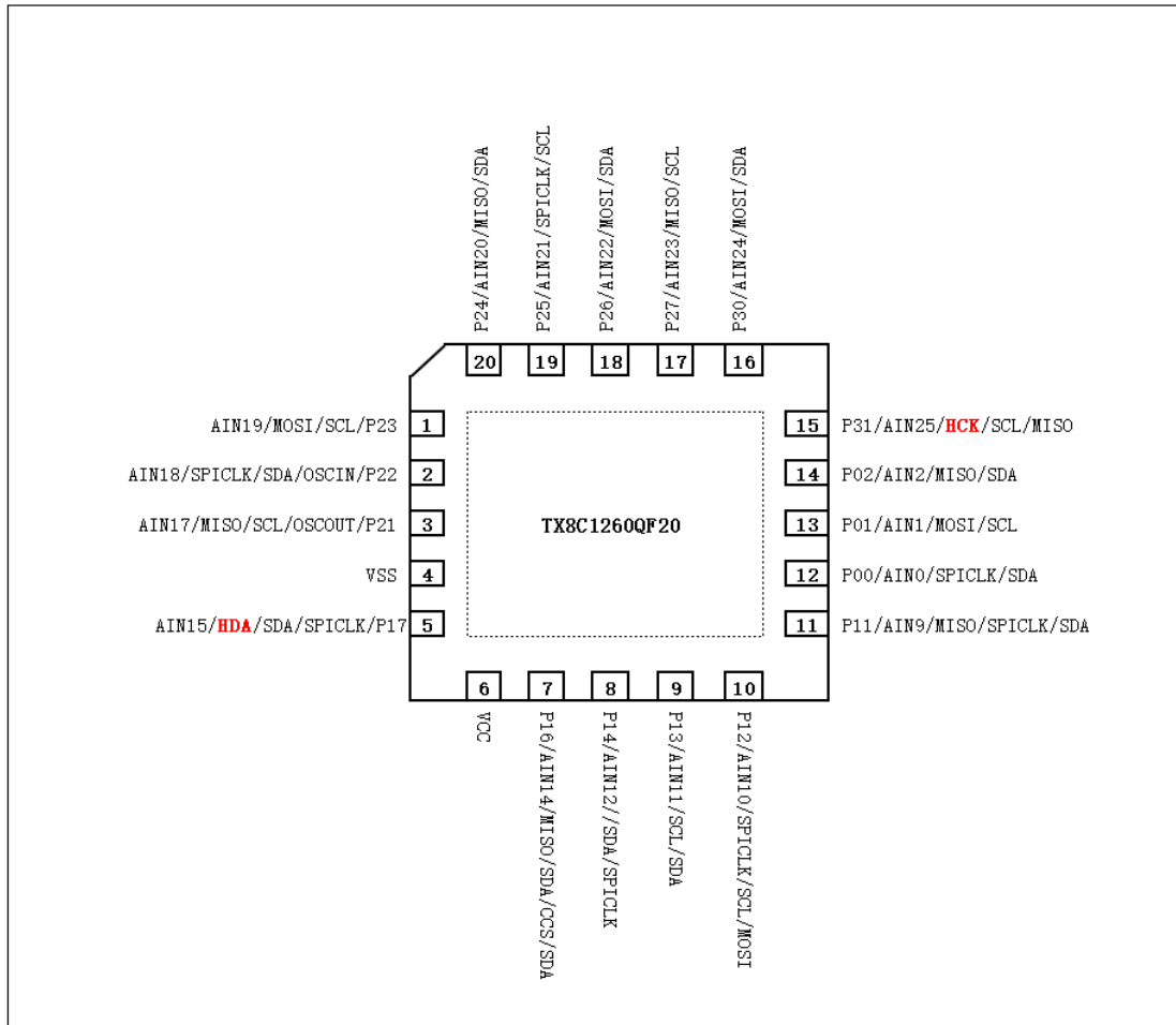
图 3 - TX8C1260QF20 (QFN20) 封装图
