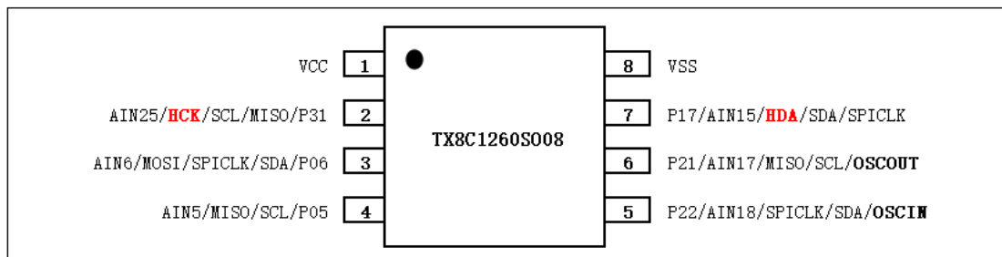
图 4 - TX8C1260S008 (SOP8) 封装图
