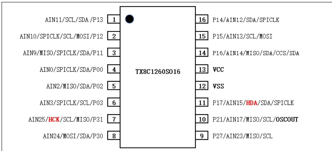
图 6 - TX8C1260S016 (SOP16) 封装图
