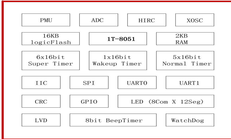
图 1 - TX8C1260 功能结构图
