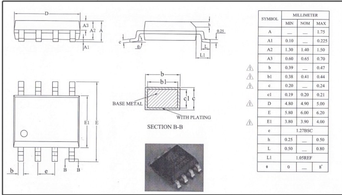
图 9- SOP8 封装 POD 图
