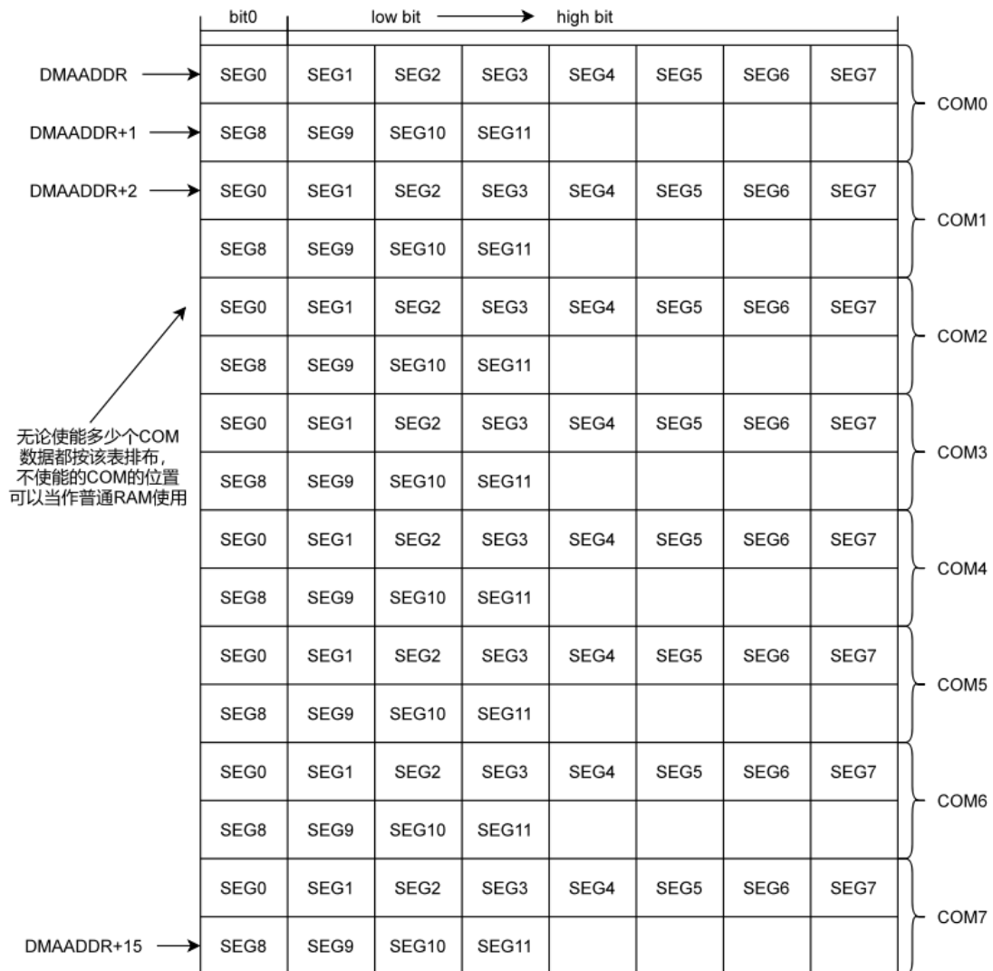
图 22-2 COM 扫描的数据结构
