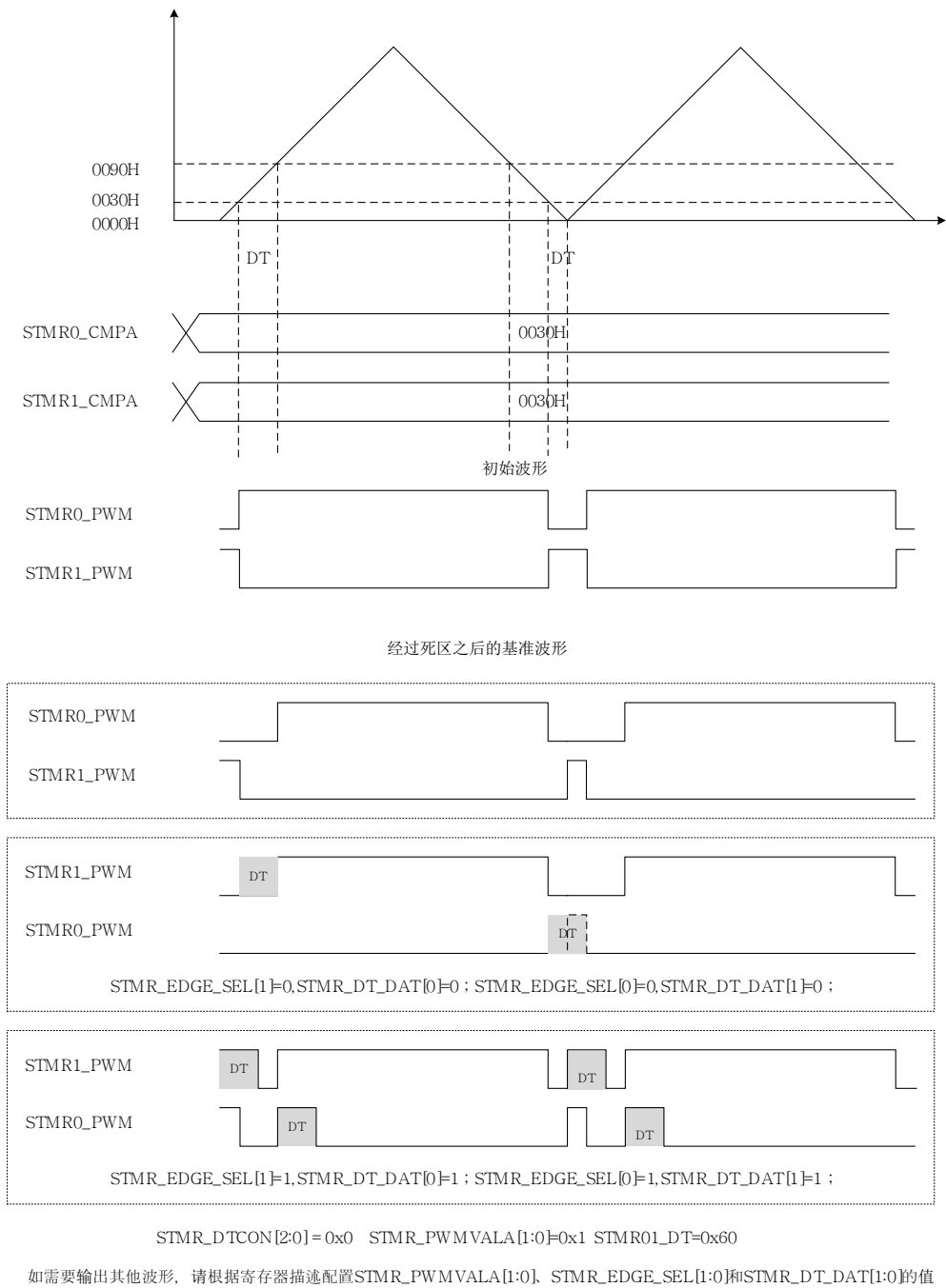
图 16-17 死区模式 0 占空比值减死区小于零时互补波形图 2
