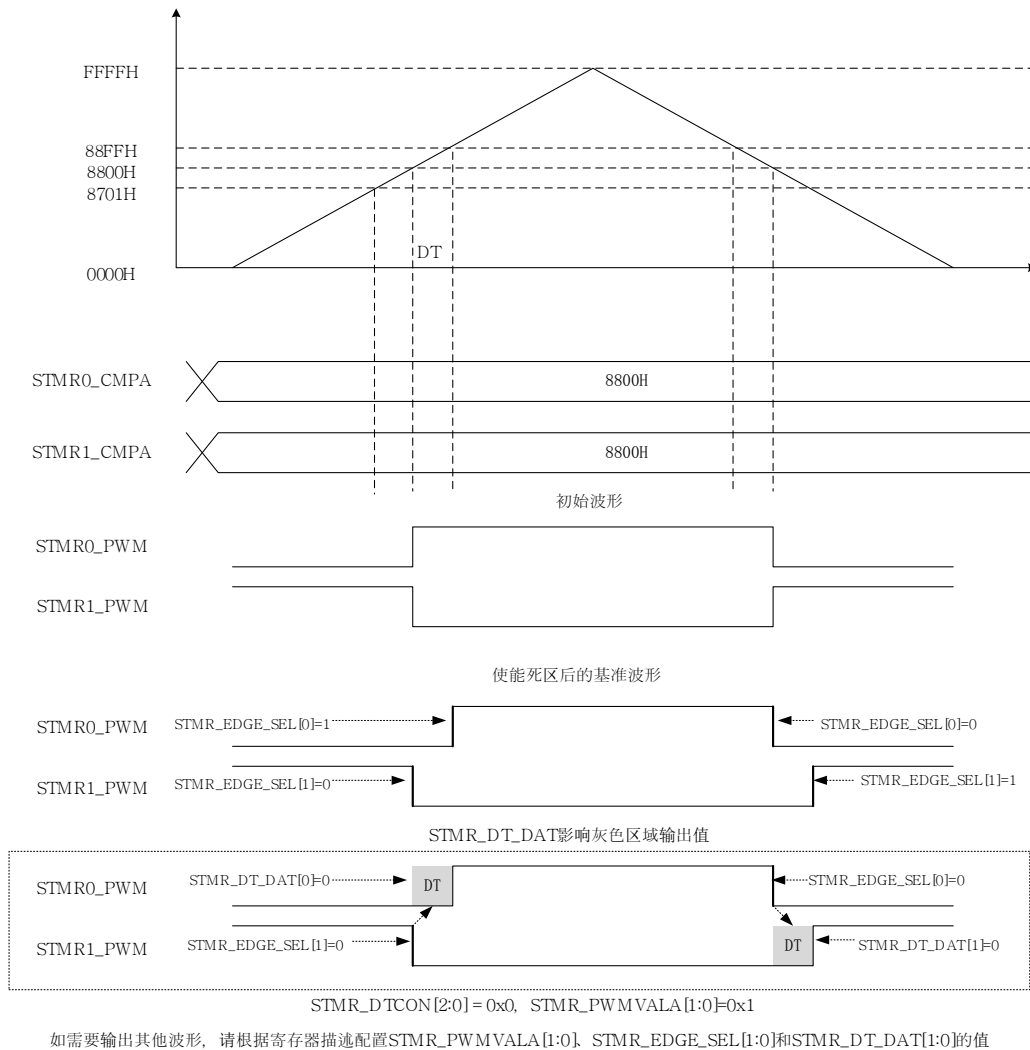
图 16-15 死区模式 0 互补波形图
