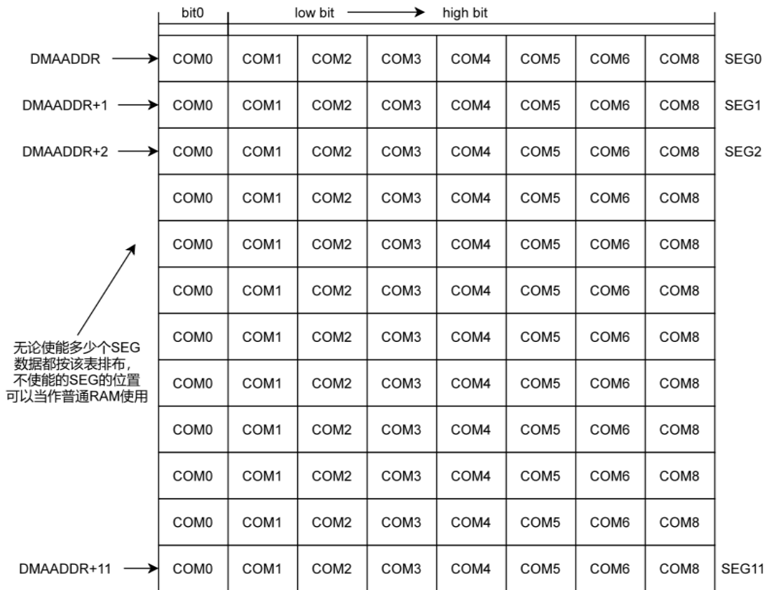
图 22-3 SEG 扫描的数据结构
