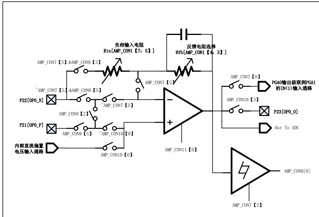
21-1 运放 PGA0 电路结构框图
