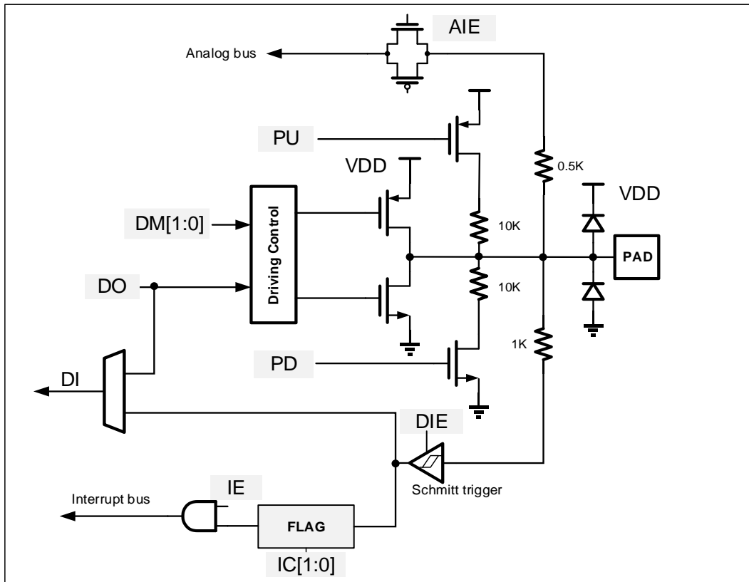
图 9-1 IO 结构图
