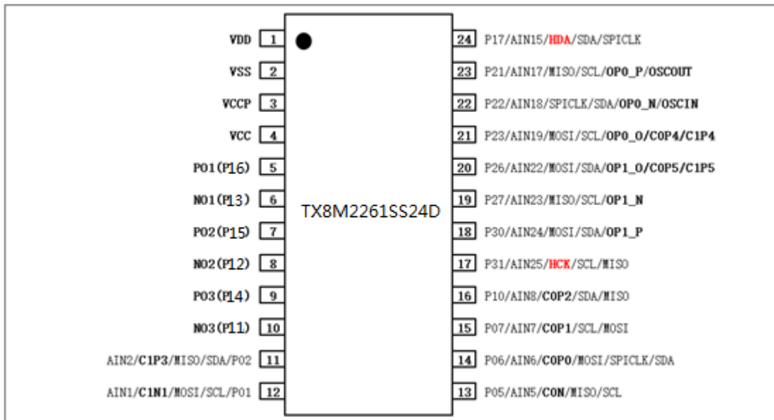
图 2 - TX8M2261SS24D (SSOP24) 封装图
