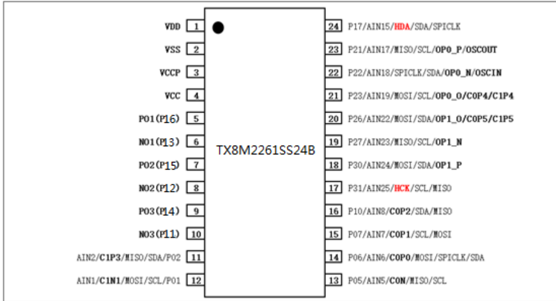
图 1 - TX8M2261SS24B (SSOP24) 封装图
