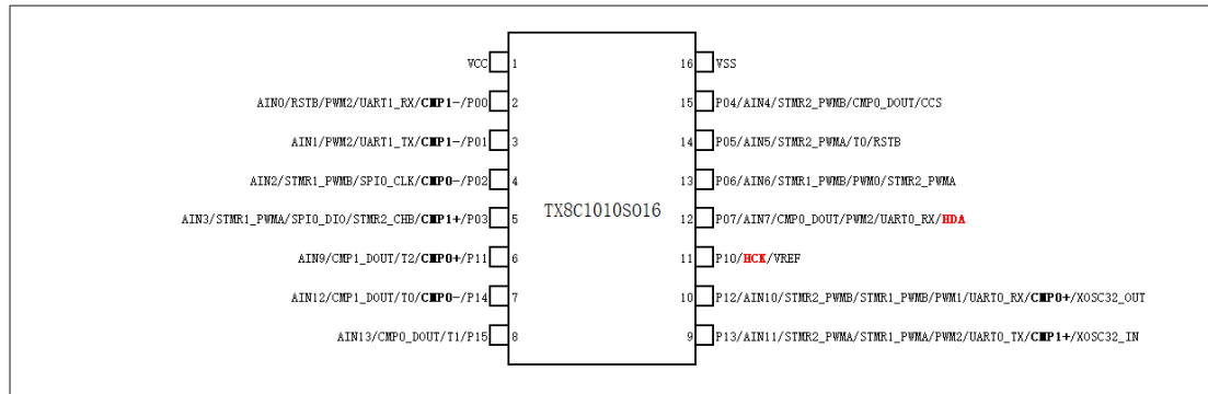
图 1-4 TX8C1010S016 (SOP16) 引脚图
