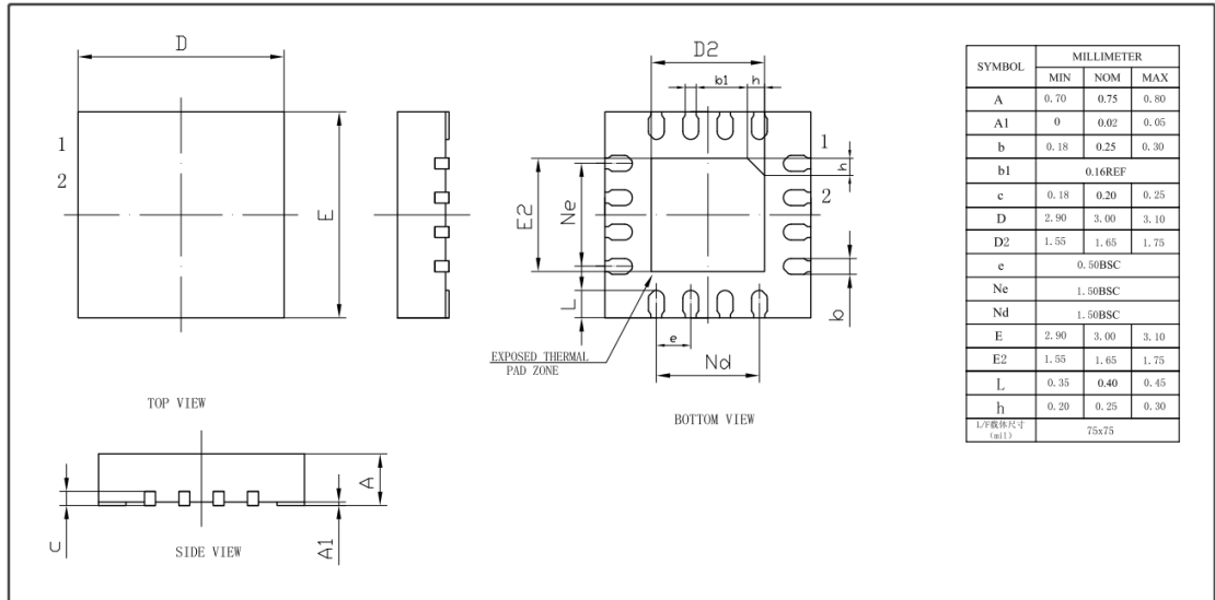
图 1-10 QFN16 封装 POD 图
