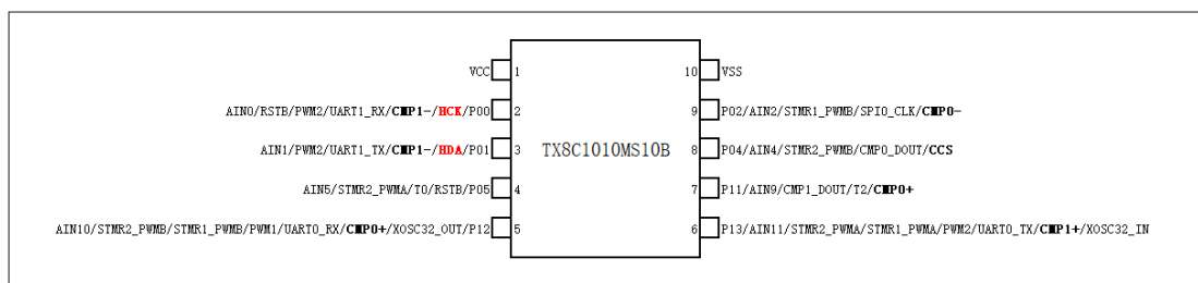
图 1-2 TX8C1010MS10B（MSOP10）引脚图
