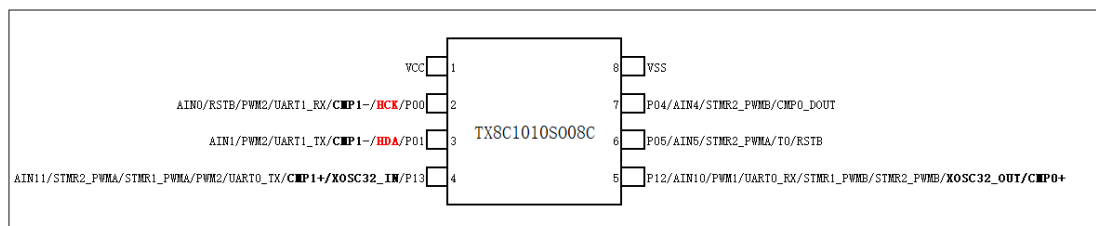
图 1-1 TX8C1010S008C（SOP8）引脚图
