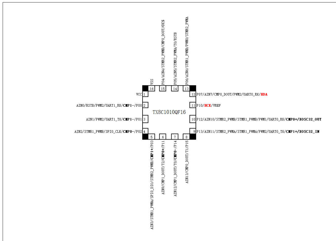
图 1-5 TX8C1010QF16 引脚图
