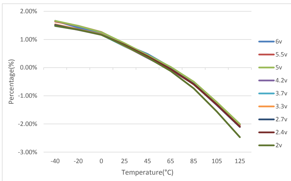
图 2-3 HIRC 全温度范围偏差百分比
