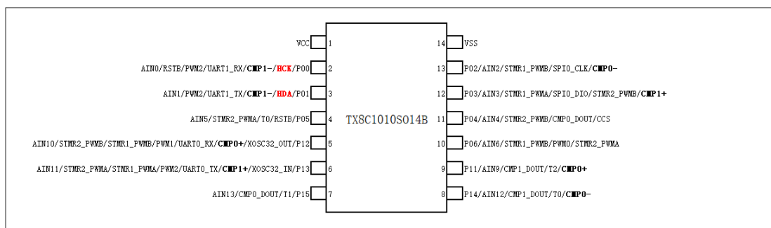
图 1-3 TX8C1010S014B（SOP14）引脚图
