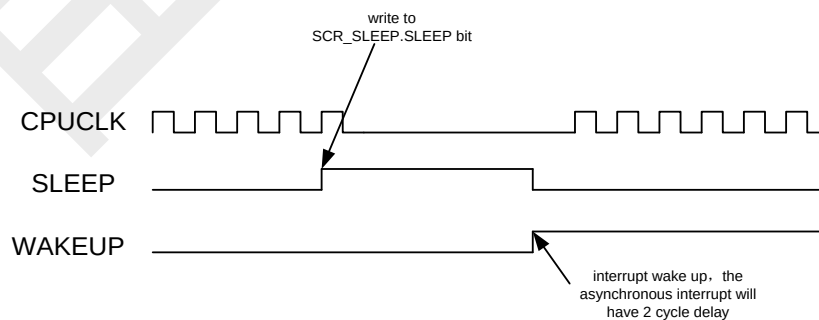
图 11-1 睡眠模式休眠和唤醒时序图
