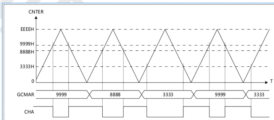
图 10-9 PWM 输出示意图
