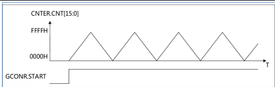
图 10-3 计数模式示意图
