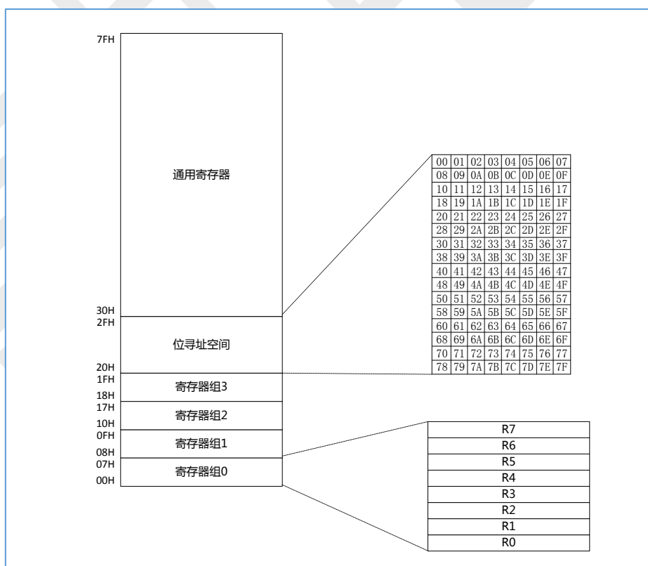
图 6-3 内部低 128 字节数据空间分配
