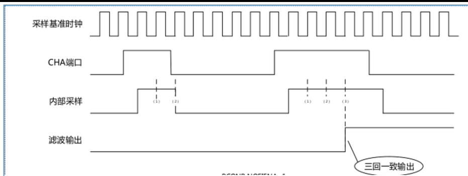
图 10-6 数字滤波示意图
