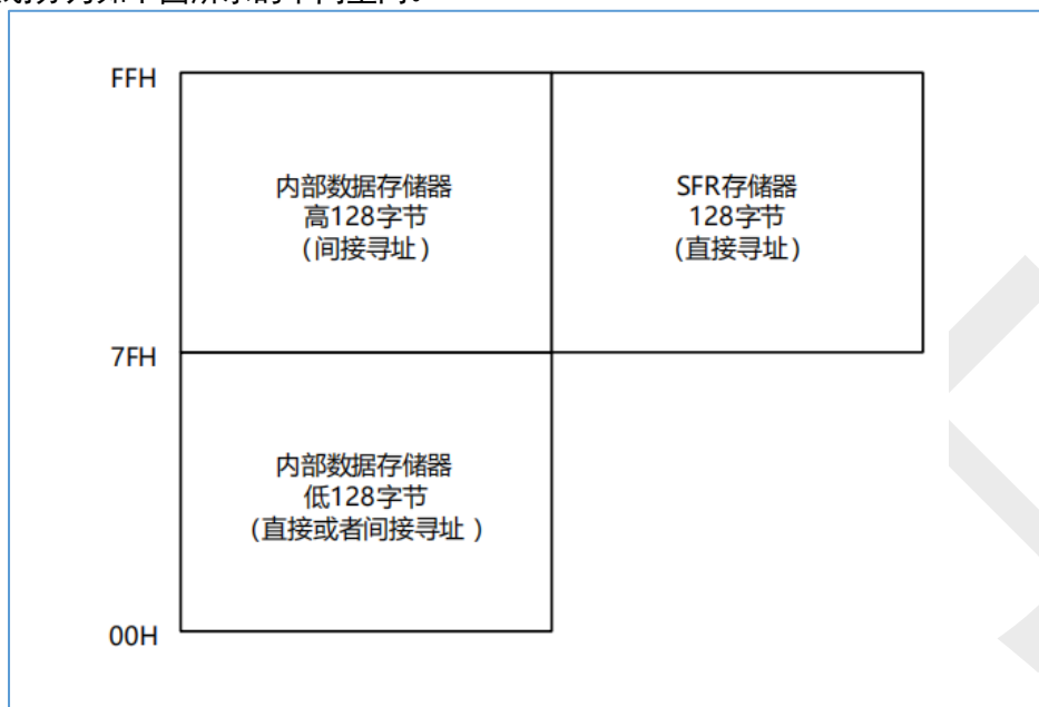
图 6-2 数据存储器
