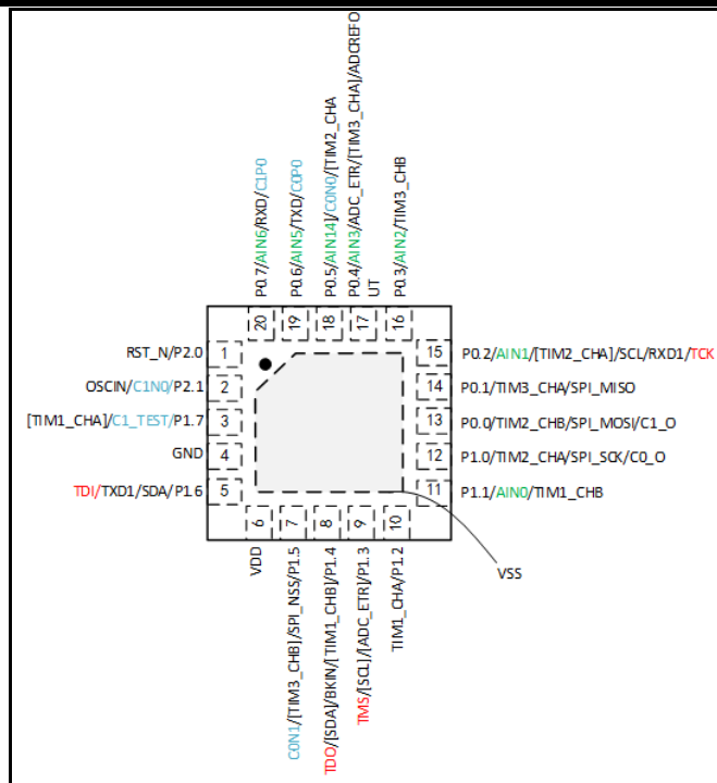
图 3-3 RC6F9003EB (QFN20) 封装脚位图
