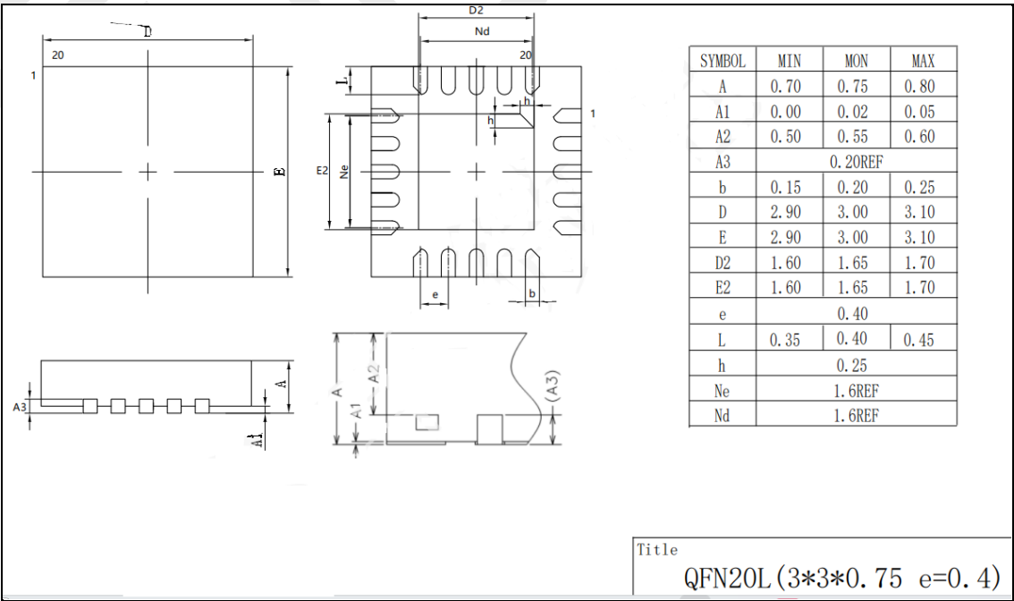
图 16-2 QFN20 封装外形图
