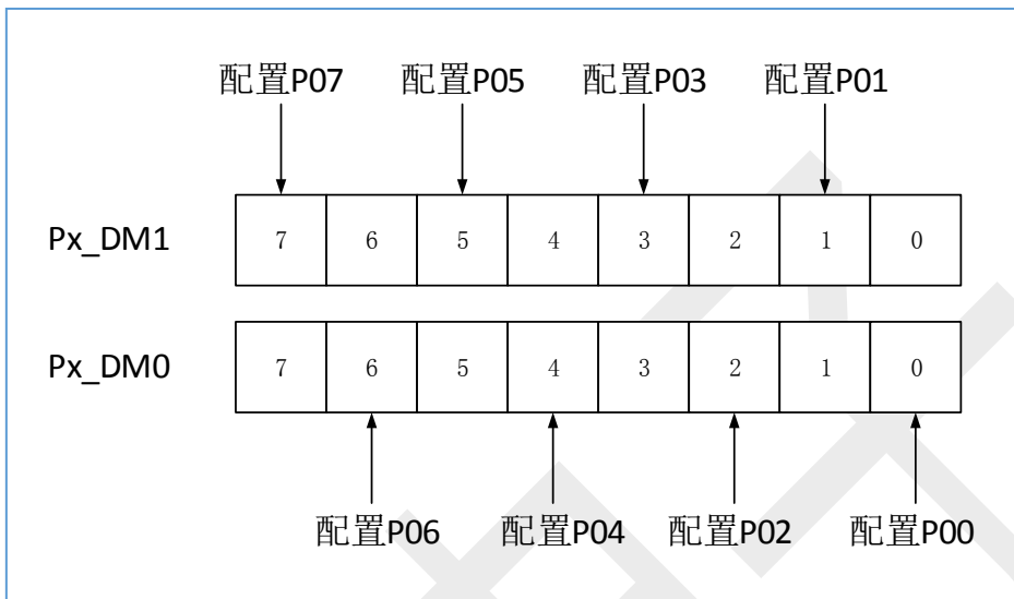
图 4-2 I/O 配置图
