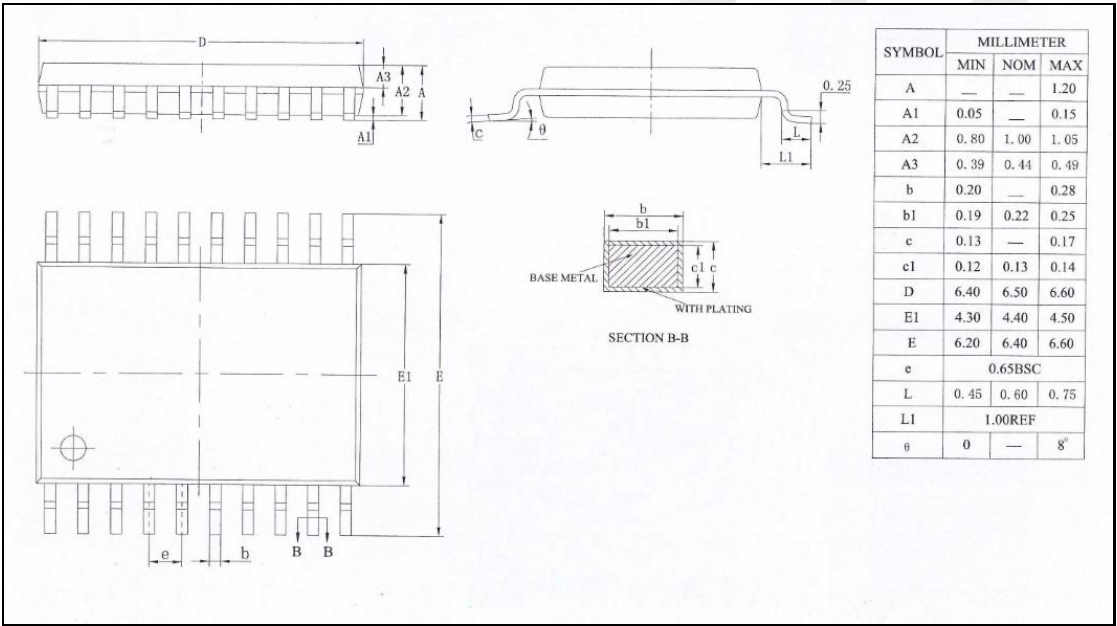
图 16-1 TSSOP20 封装外形图
