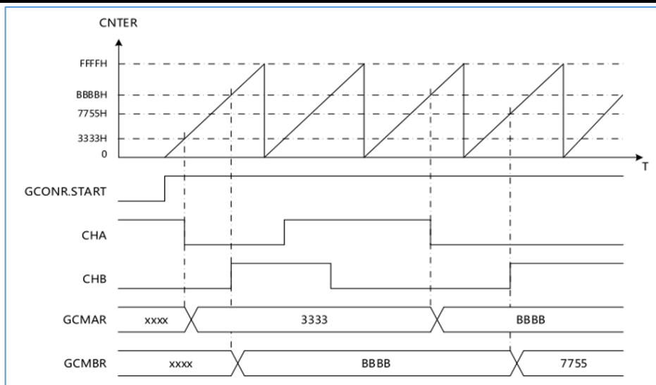
图 10-5 捕获模式示意图
