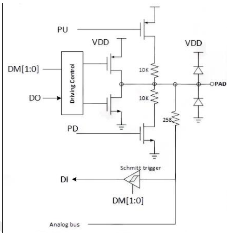
图 4-1 GPIO 结构图
