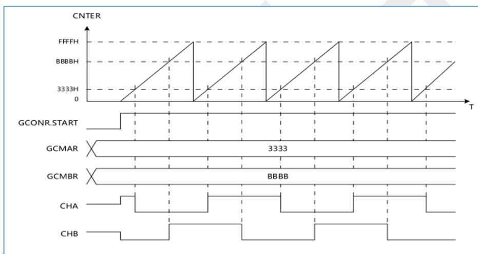
图 10-4 比较输出示意图
