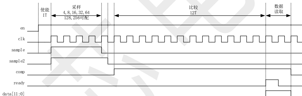
图 10-4 ADC 时序图
