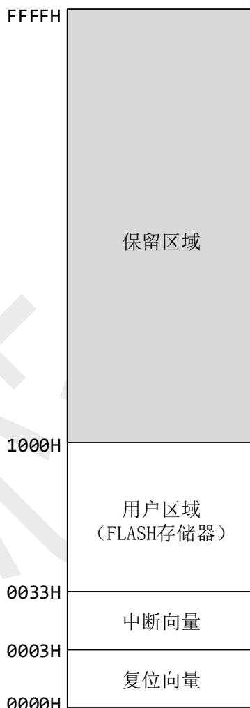
图 2-1 程序存储空间
