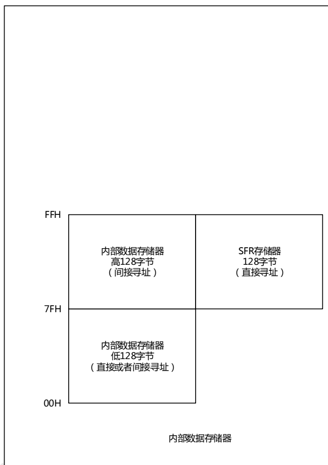
图 6-2 数据存储器
