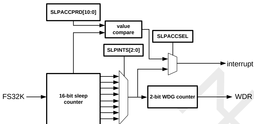
图 11-3 看门狗定时器
