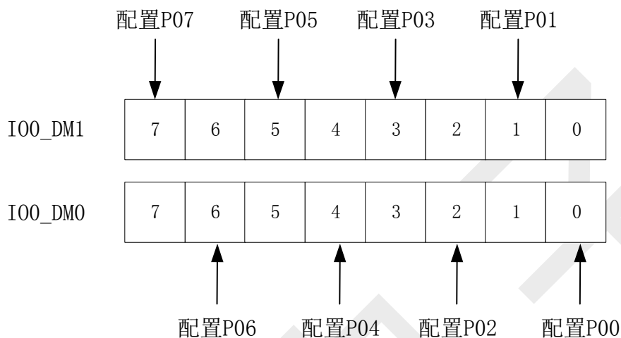
图 4-3 I/O 配置图
