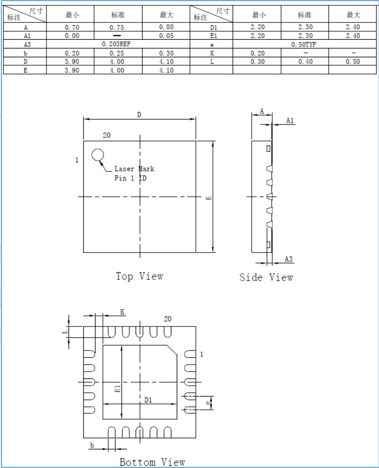
图 15-2 QFN20 封装外形图
