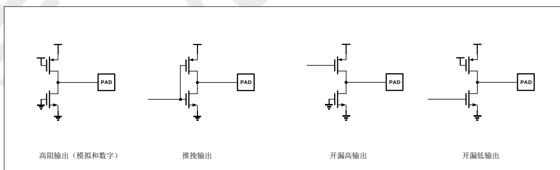
图 4-4 GPIO 驱动模式
