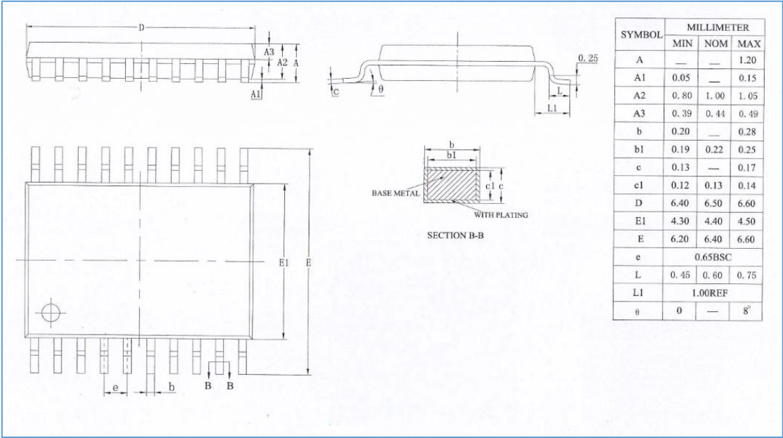
图 15-1 TSSOP20 封装外形图
