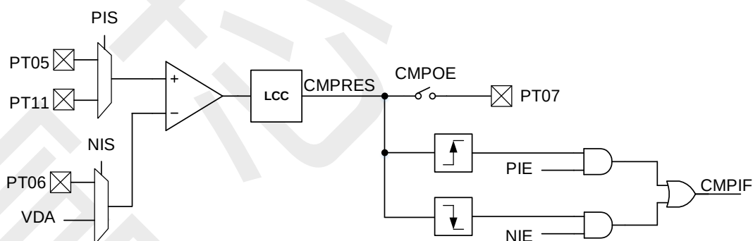
图 10-17 比较器 0 电路结构框图
