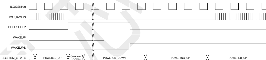
图 11-2 深度休眠唤醒时序
