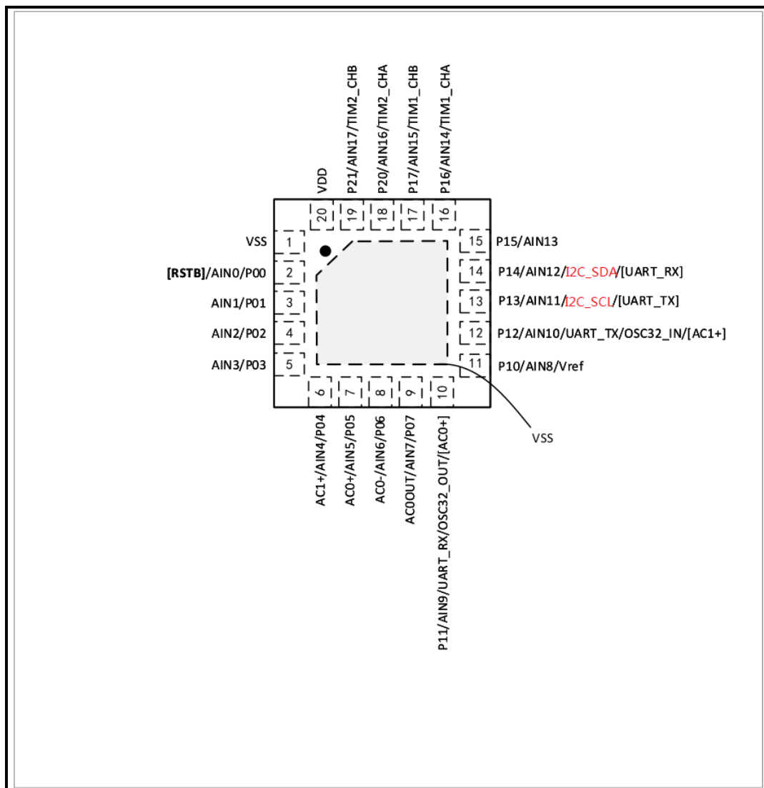
图 3-4 RC6F8001EB (QFN20)引脚图
