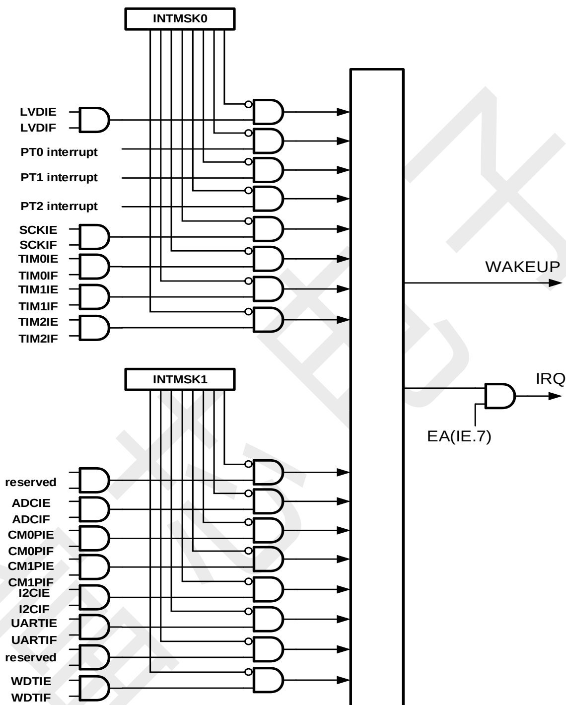
图 7-2 中断结构框图
