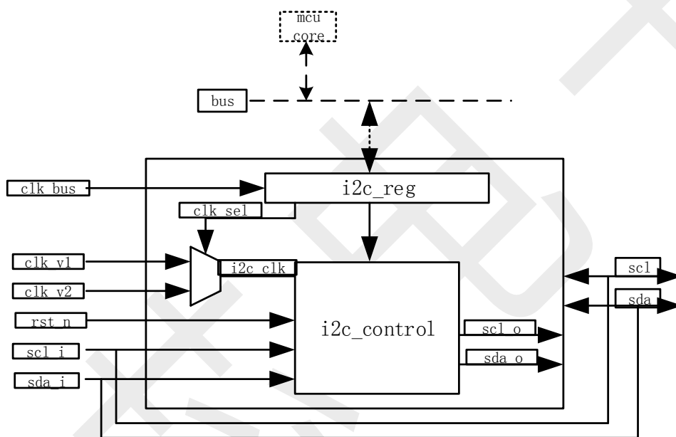
图 10-14 I2C 结构框图
