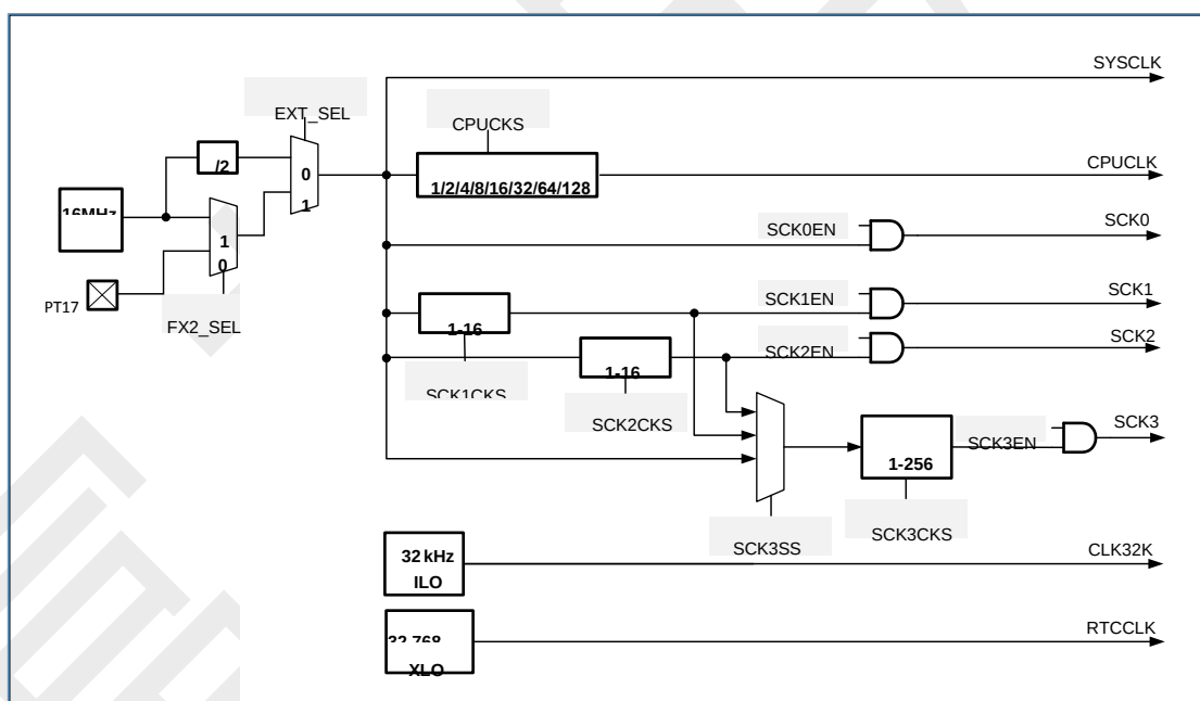
图 8-1 时钟结构框图
