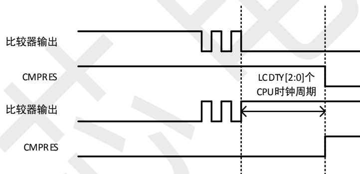
图 10-5 比较器数字滤波功能
