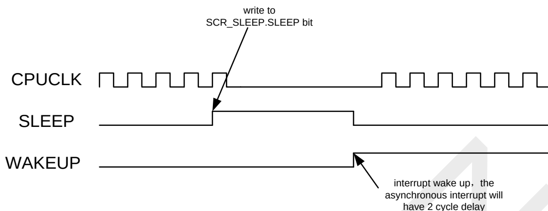
图 11-1 睡眠模式休眠和唤醒时序图
