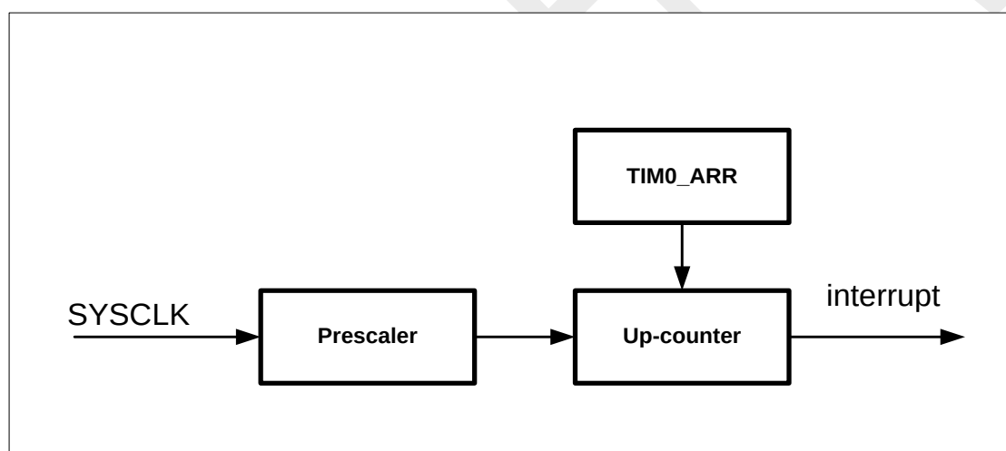
图 10-1 TIMER0 结构框图
