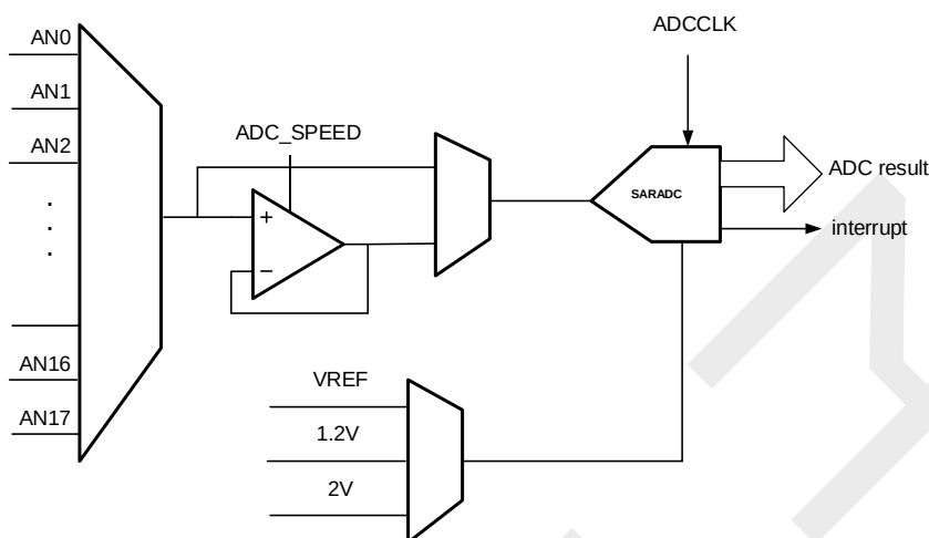
图 10-3 ADC 结构框图
