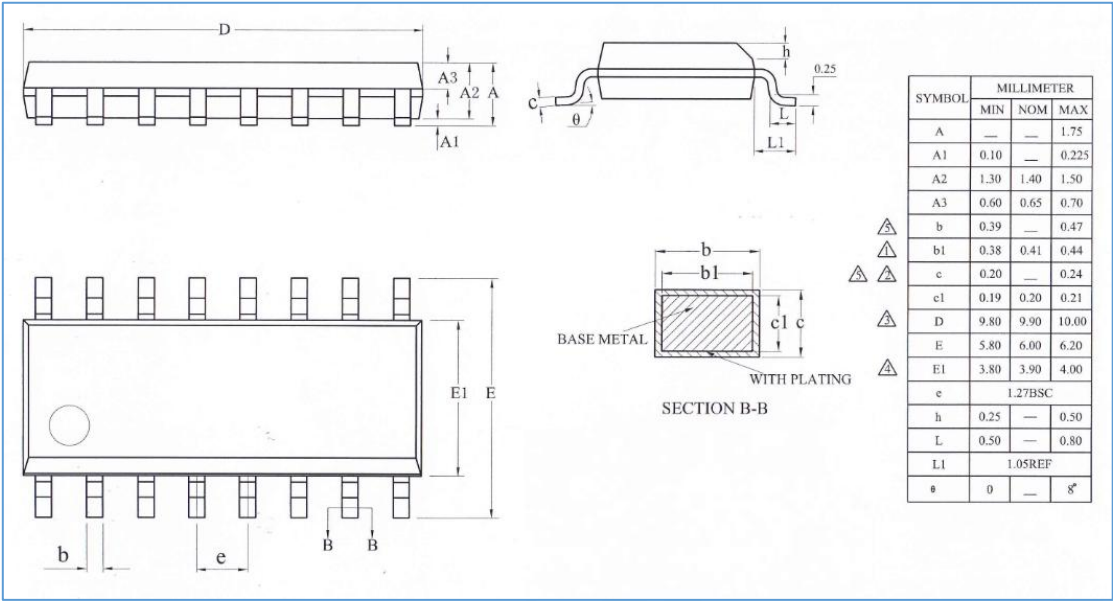
图 15-3 S0P16 封装外形图
