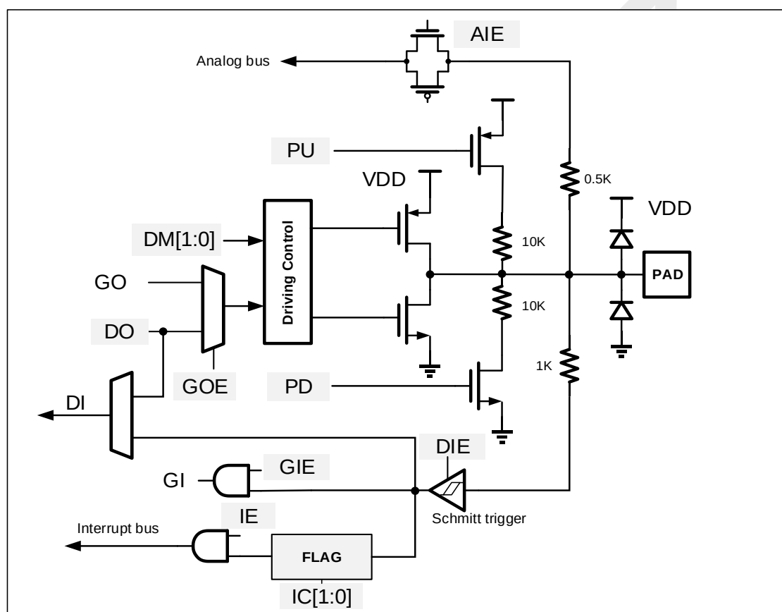
图 4-1 GPIO 结构图
