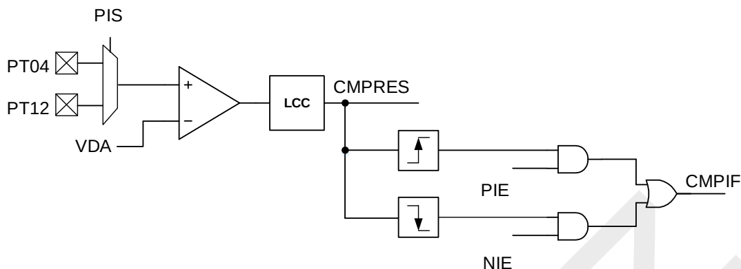
图 10-18 比较器 1 结构框图
