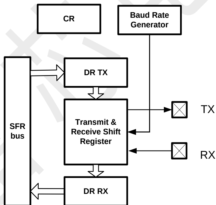
图 10-13 UART 结构框图
