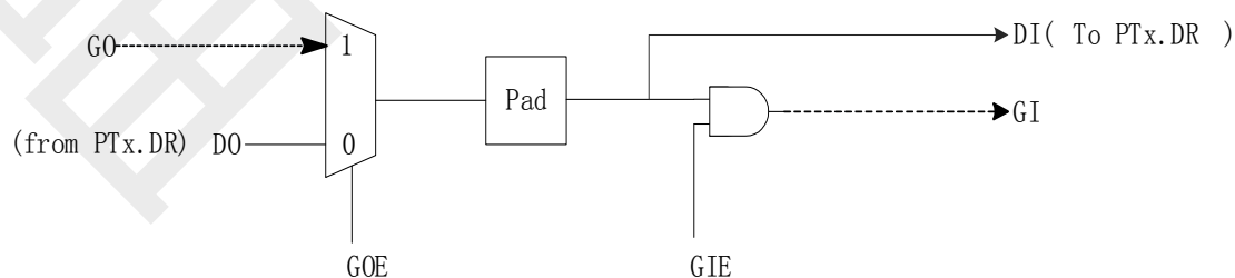
图 4-2 GPIO 复用结果说明
