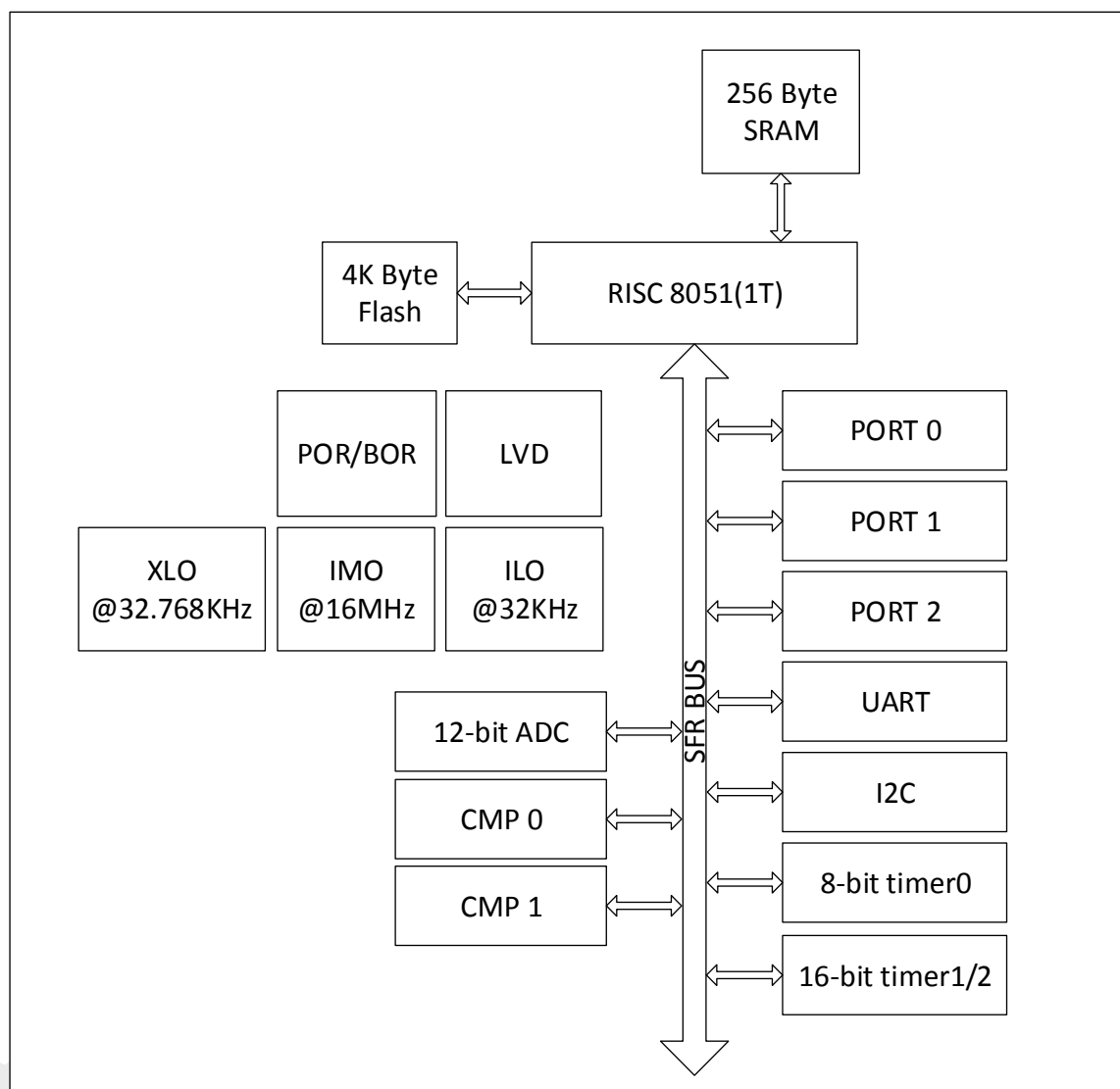
图 3-1 系统功能结构框图
